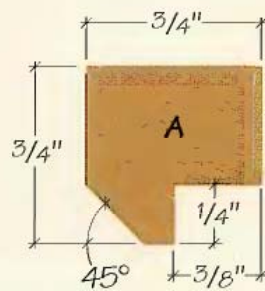
DETAIL: FRAME
