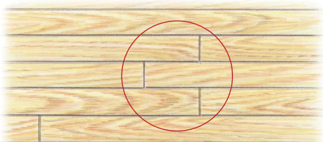
H-pattern
