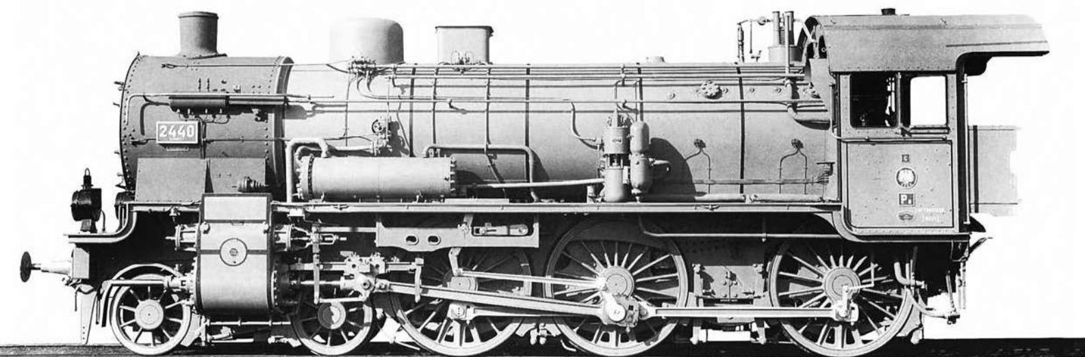
Diese P 8 wurde 1915 als 2440 Hannover von Schwartzkopff gebaut und verfügte über einen Knorr-Oberflächenvorwärmer und eine Knorr-Kolben-seispumpe. An der Rauchkammer ist zudem der Automat zum Schließen der Überhitzerklappen erkennbar. Foto: Archiv Michael Meinhold
