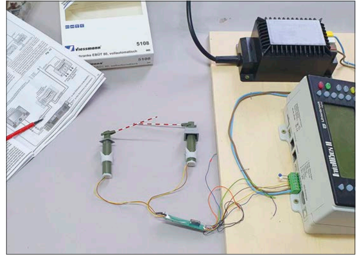
In der Praxis kann man die Viessmann-Schranken (z.B. # 5108 ) mit dem zugehörigen Digitaldecoder zuerst einmal an eine Digitalzentrale (IB2-Gleis Ausgang) anschließen und sie über das Magnetartikelm Menü mit den Tasten zum Testen schalten und die Adresse ändern.
