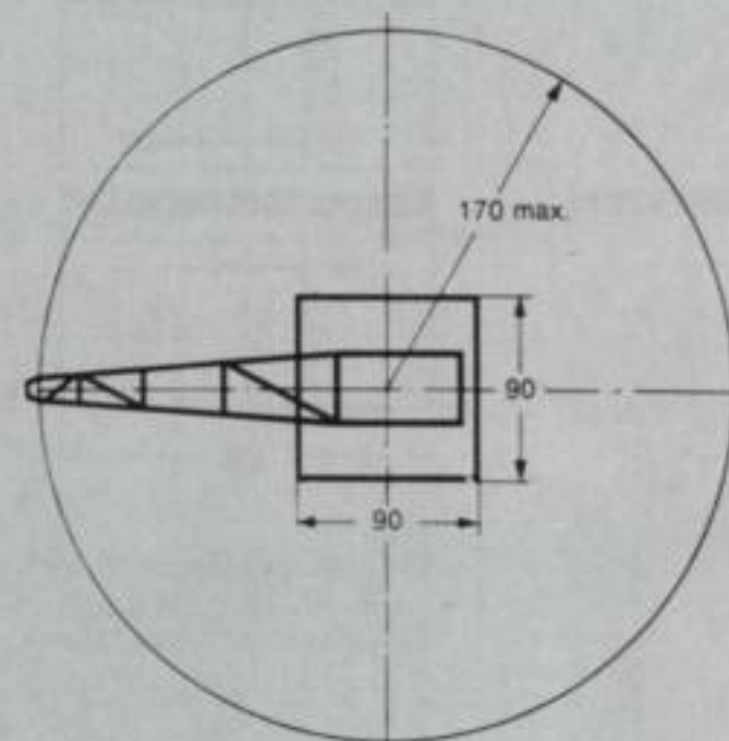
7051 Ferngesteuerter Drehkran
