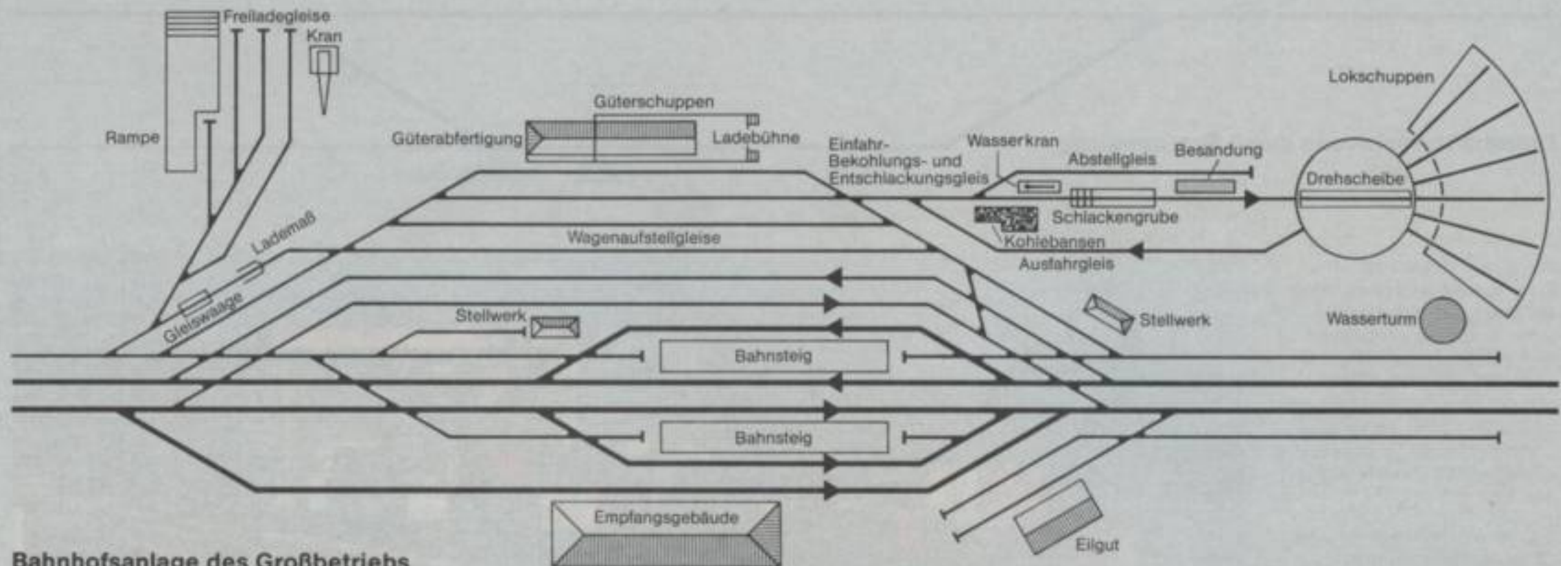
Bahnhofsanlage des Großbetriebs
