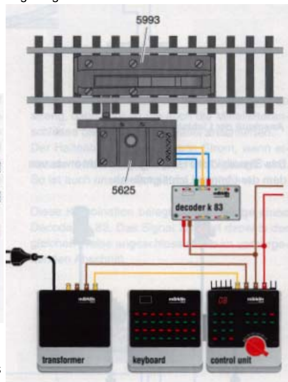
Spur 1- Entkupplungsgleis 5993
