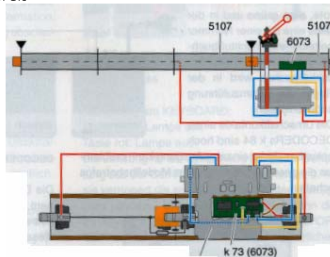
Signal- Grundplatte
