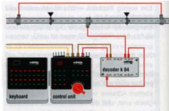
Der Decoder k 84 als Signalersatz
