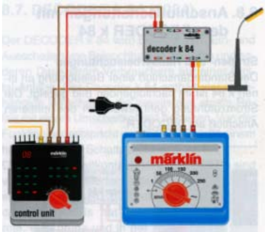
Der Decoder k 84 als Signalersatz
