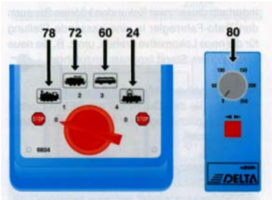
Digital-Adressen der DELTA-Lokomotiven
