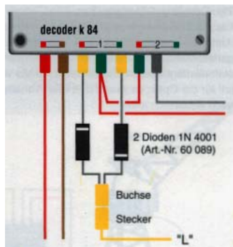
Anschluß der Schiebebühne 7294 über einen Decoder k 84
