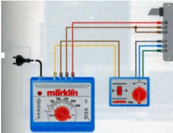
Anschluß der Drehscheibe 7286 bei konventionellem Fahrbetrieb
