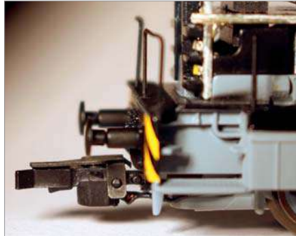
Für den Umbau der TT-106 wurde eine Digitalkupplung von SD-Modellbau verwendet.
