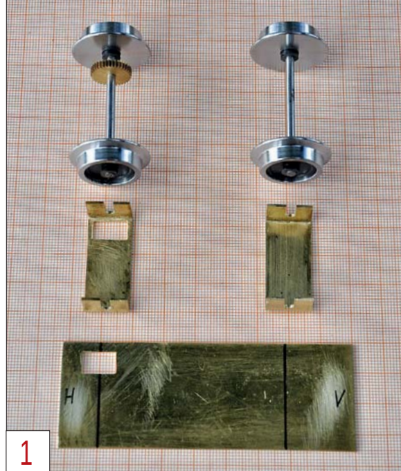
1 Der Fahrschemel des Modell-Trabis sowie die Achshalterbügel wurden aus ein Millimeter starkem Messingblech angefertigt.
