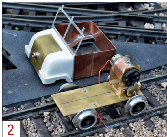
2 Im noch unlackierten Zustand wurde das Eigenbaumodell einer ausgiebigen Fahrerprobung auf der Freilandanlage unterzogen.
