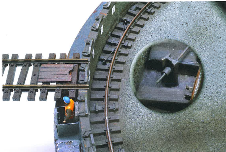
Auch die 40 Winkel, welche die Schwellen des Laufkreises sichern, bildete Vollmar detailtreu nach. Das kurze Schienenstück des Laufkreis-Ankers, das man in der Vergrößerung erkennt, ist ein TT-Profil!
