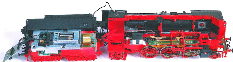
Bewährte Antriebskonzeption: Tendermotor mit Schwungmasse, Kardanwelle zur Lok.
