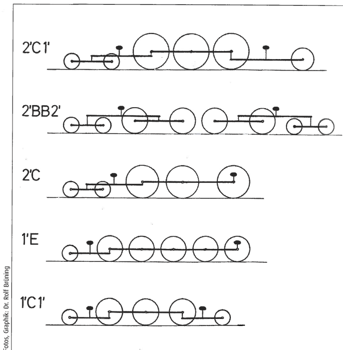
Auf einen Blick: Die Zeichnung zeigt Beispiele für die Anordnung der Führungspunkte bei verschiedenen Achsfolgen.
