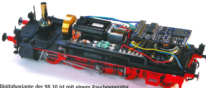
Die Digitalvariante der 98.10 ist mit einem Rauchgenerator sowie einem Lautsprecher im Führerhaus ausgestattet.
