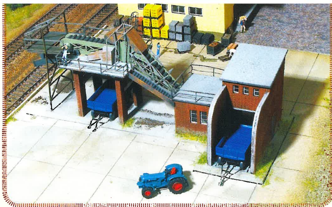
Das erste Funktionsmodell von MBZ zeigt eine Rübenverladung. Das Entladen der Hänger kann analog und digital gesteuert werden.
