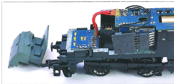
Unter dem Führerstand sind die Beleuchtungs-LED zu erkennen, rechts davor die Digitalschnittstelle.
