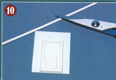
Zur Nachbildung der Türen kann man entweder Polystyrolplatten oder aber gleich noch leichter zu gravierendes Balsaholz verwenden.
