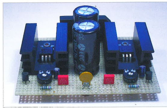
Zu Schaltbild 1: Die Platinenbestückung des symmetrischen Fahrreglers (ohne Trafo) zeigt deutlich, dass der Aufwand an Bauteilen überschaubar bleibt.
