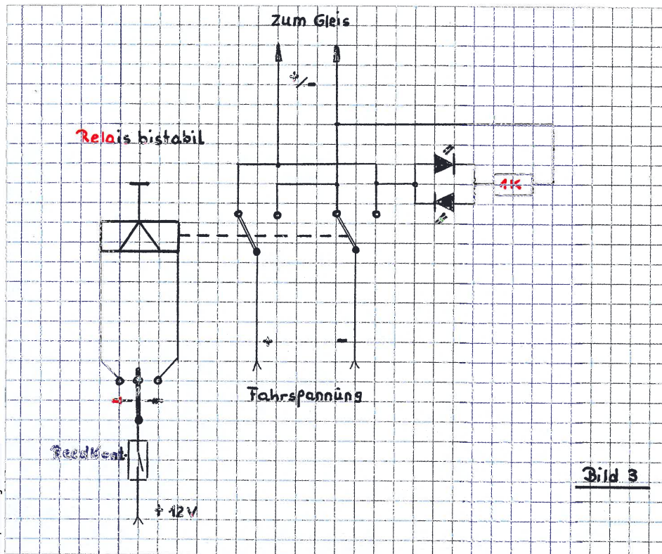
Zu Schaltbild 3: Die Schaltung für den Fahrtrichtungswechsel mit Reedkontakt und bistabilem Relais verhindert nicht nur das irrtümliche Umschalten, sondern funktioniert mit dezentralem Regelpoti gleichzeitig auch als Automatik.
