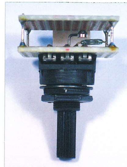
Zu Schaltbild 3: Die Schaltung für den Fahrtrichtungswechsel mit Reedkontakt und bistabilem Relais verhindert nicht nur das irrtümliche Umschalten, sondern funktioniert mit dezentralem Regelpoti gleichzeitig auch als Automatik.
