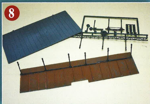
In der Zwischenzeit kommt die Überdachung des Hausbahnsteigs an die Reihe. Sie entsteht aus Auhagen-Platten und Falter-Bahnsteigstützen.
