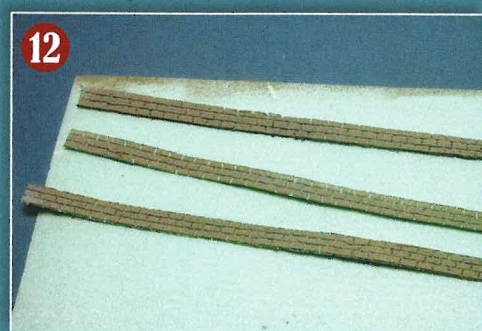
Fertig graviert, koloriert und auf passendes Maß geschnitten sind die Sockelumrandungsstreifen bereit zur Verklebung auf den EG-Außenwänden.
