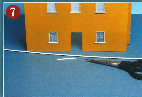
Erst muss die Farbe gänzlich getrocknet sein, ehe man darangehen kann, sich mit der Anbringung der umlaufenden Sockelmauer zu beschäftigen.
