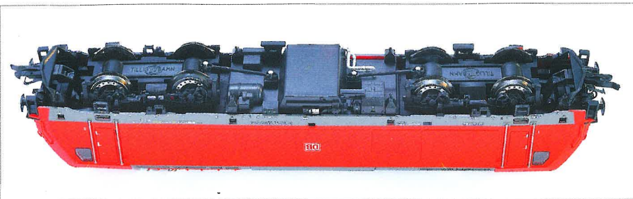
Der Blick unter die Lokomotive ist lohnenswert. Dort sind unter anderen die nachgebildeten Zug- und Druckstangen zu erkennen.
