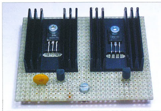
Passend zu Schaltbild 1: Das Innenleben des Handreglers mit Mittelstellung (siehe auch Bild lks.) ist recht einfach aufzubauen und einzusetzen.
