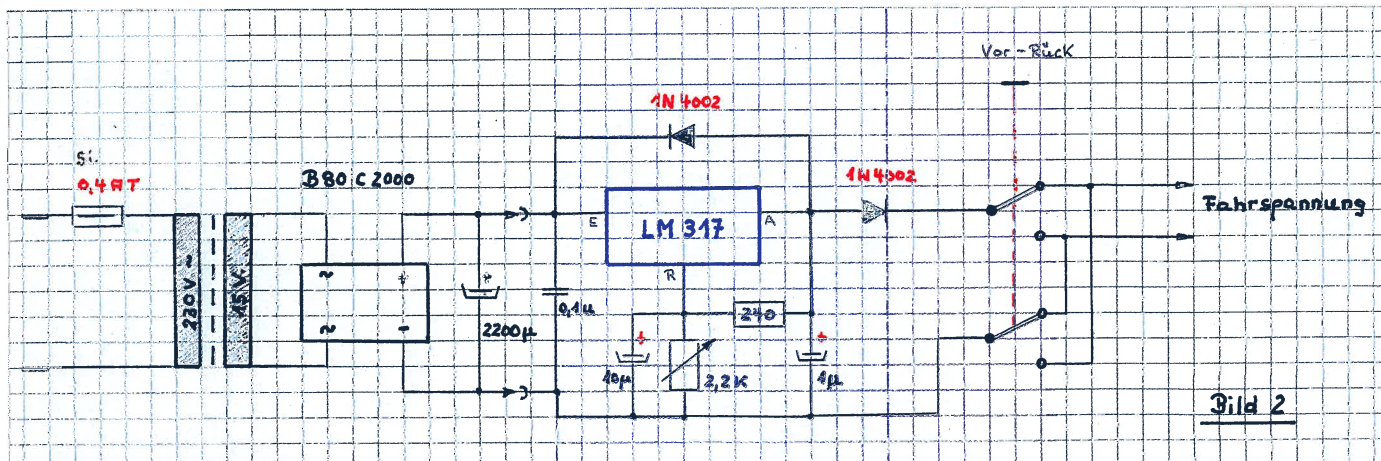
Schaltbild 2, Fahrregler mit Richtungsumschalter: Die Spannungsversorgung besteht aus einem passenden Transformator, dem zugehörigen Gleichrichter samt Lade-Elko. Diese Komponenten können wie auch der komplette Fahrregler separat unter der Anlage angebracht werden.
