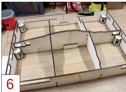
6 Der fertige Rahmen für „Oberschirma“: Die beiden Segmente weisen jeweils zwei Zwischenspannten zur Stabilisierung auf.
