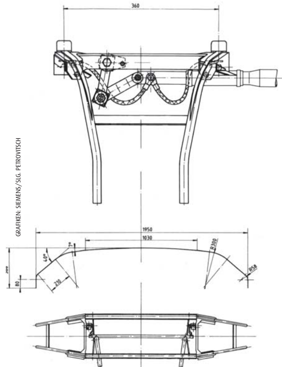
Detaildarstellung der DB-Palette mit doppelten Auflaufhörnern. Die vertikal und horizontal federnde Halterung an der Scheitelrohrwelle erfolgt über winkelelastische Lenker.
