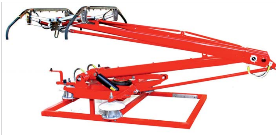
Der ATR 95 für den HG-Zug ETR 500 der FS macht das Gelenkviereck evident, das den gefächerten Oberteil in Stellung hält. Am Palettenkopf sind die gefederten und gedämpften Schwingen der Schleifstückhalterungen ersichtlich, unter dem Basisholm erkennt man den Luftfederbalgantrieb.
