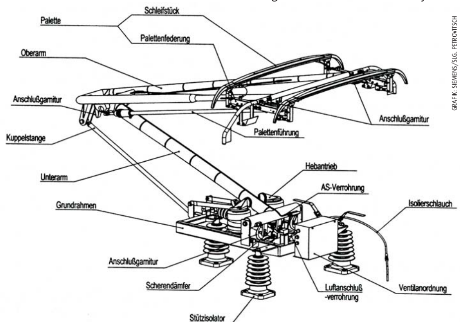
Der ATR 95 für den HG-Zug ETR 500 der FS macht das Gelenkviereck evident, das den gefächerten Oberteil in Stellung hält. Am Palettenkopf sind die gefederten und gedämpften Schwingen der Schleifstückhalterungen ersichtlich, unter dem Basisholm erkennt man den Luftfederbalgantrieb.
