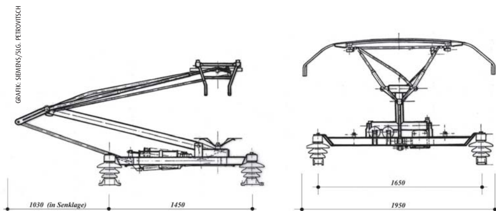
Übersichtszeichnung des Standard-Einholmbügels der DB in der Bauform SBS 81 mit Vierpunktbasis (Aufstandspunkte wie DBS 54) und Kolbenantrieb auf Hochspannungspotential, verwendbar unter anderem für 103, 111, 120 und 151.
