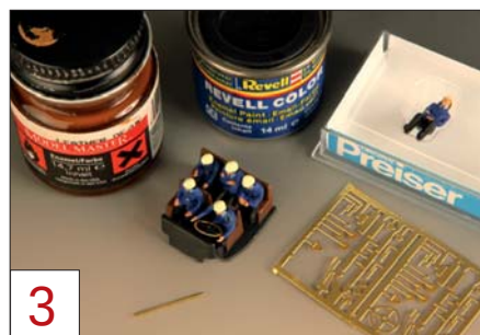
3 Das Führerhaus-Innere wird nach der farblichen Gestaltung mit einem Weinert-Lenkrad und mit Personal von Preiser bestückt.
