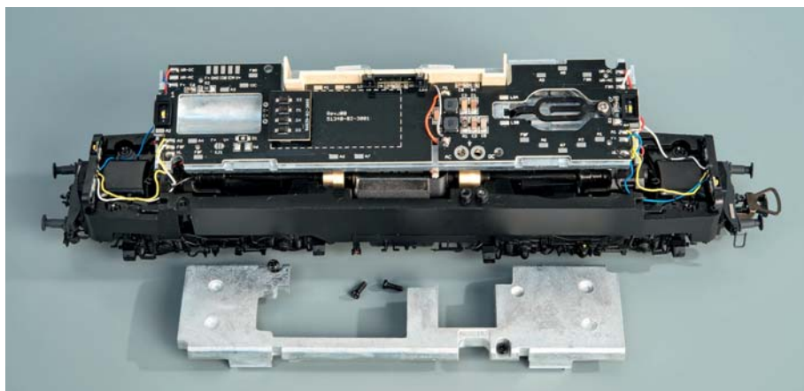
Das typische Innere einer modernen H0-Lokomotive. Alles ist aufgeräumt und konstruktiv für eine digitale Aufrüstung vorbereitet.
