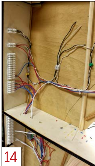
Die Verkabelung ist konventionell: Die Leitungen sind mit Heißkleber fixiert und werden über Lüsterklemmen geführt. Unten ist ein kompakter MTB-Weichenantrieb zu erkennen.
