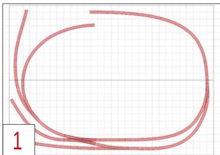
1 Die sichtbare Streckenführung besteht aus einer Hälfte der „verschlungenen Acht“. Drei Abstellgleise bieten Rangiermöglichkeiten.
