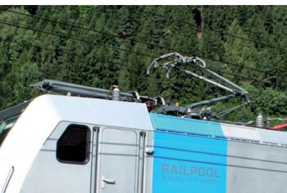
Stromabnehmer DSA 200 aus Entwicklung Dornier beziehungsweise Produktion Sternmann auf der Traxx 186 108 von Railpool mit Gleichstrom-Palette für Italien.
