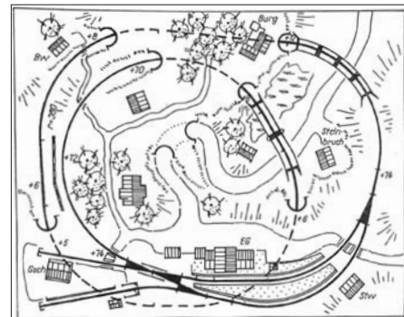
Als Inspiration diente dieser alte Gleisplan.
