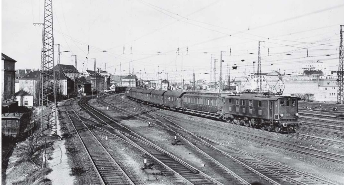
Auch eine Art S-Bahn: E5233 verlässt den Bahnhof Nürnberg am 18. April 1955 mit dem abendlichen Pendlerzug P 1137 nach Lichtenfels.
