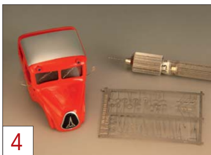
4 Das Äußere wird durch angesetzte Scheibenwischer und Spiegel aus einem Zurüst-Satz von Weinert aufgewertet.
