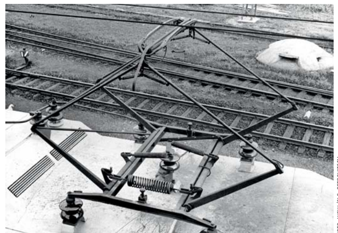
Mit der Bauart IV (Firmenbezeichnung WVSS 51) führten die ÖBB 1951 bei den Neubaureihen 1040 und 1041 den Einbügel-Betrieb ein.
