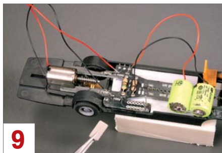
9 Nach dem Einlöten der Bauteile und dem Einkleben des Motors erfolgt ein erster Test des Antriebs.
