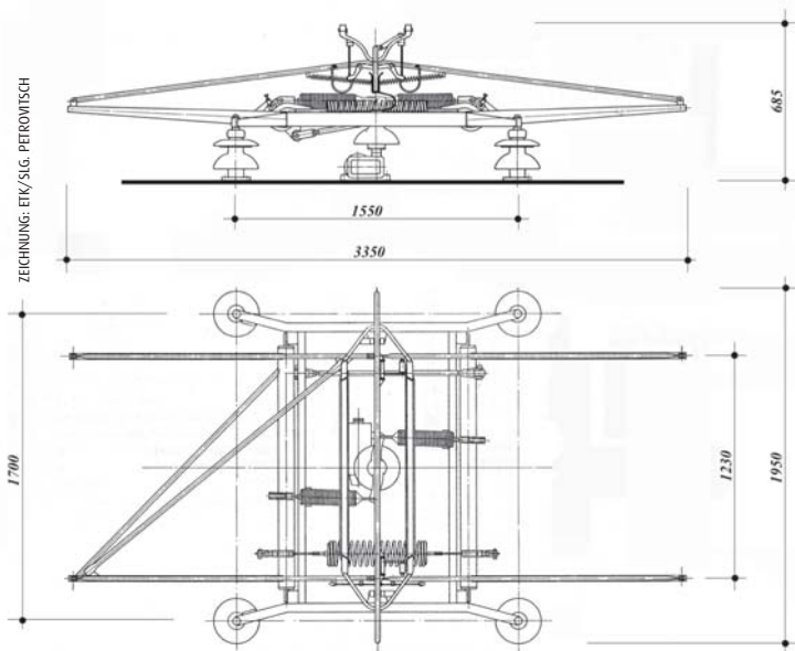
Zusammenstellungszeichnung des ab 1955 auf den ÖBB-Neubauloks verwendeten Scherenstromabnehmers Bauart V (Siemens WVSS 54).
