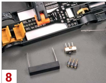
8 Für die elektrischen Komponenten müssen noch diverse Aussparungen im Unterboden geschaffen werden.
