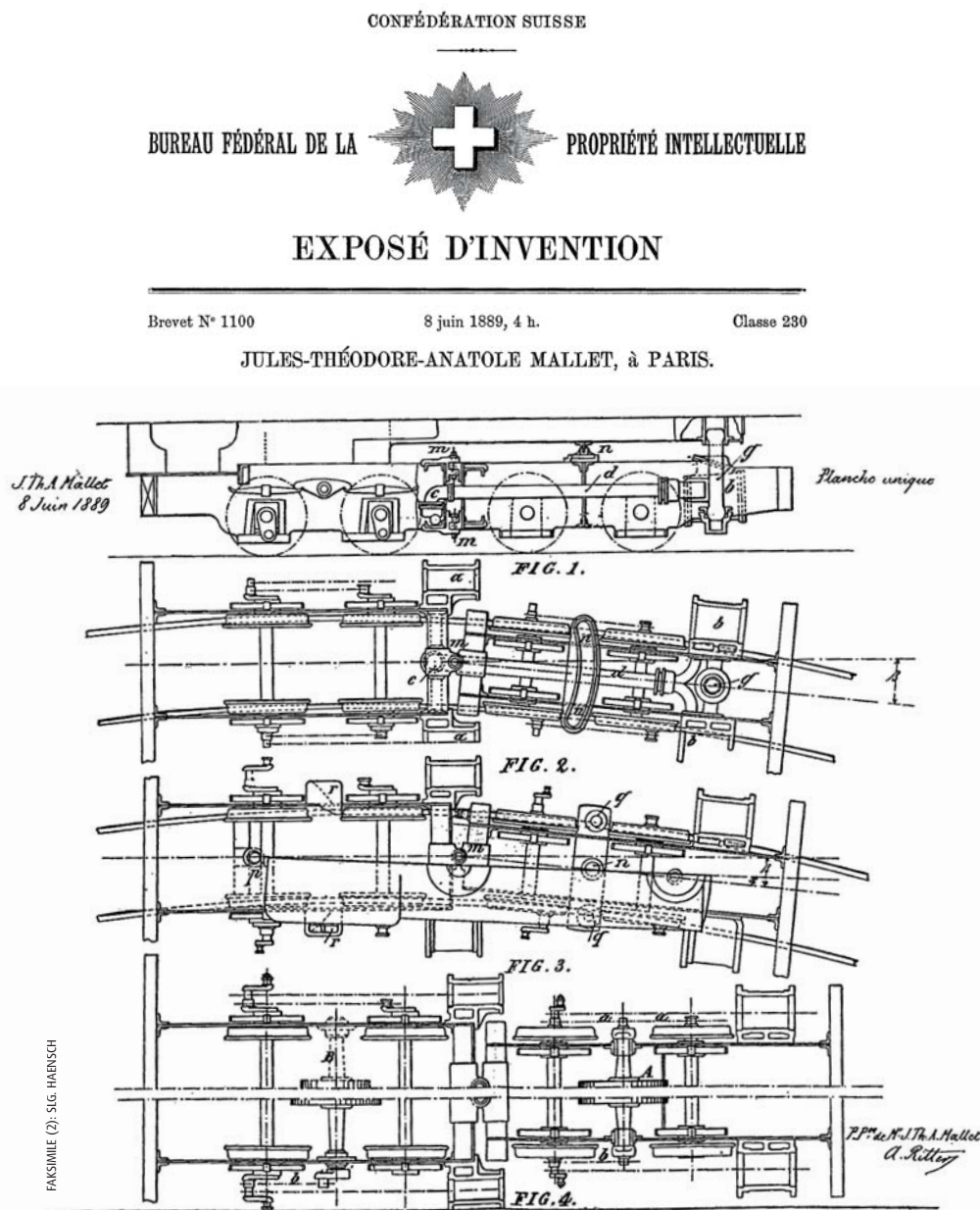
Die Schweizer Patentschrift von 1889 zeigt deutlich das Prinzip und die typischen Merkmale der ersten Mallet-Lokomotiven, etwa den Innenrahmen vorn und einen Außenrahmen hinten.
