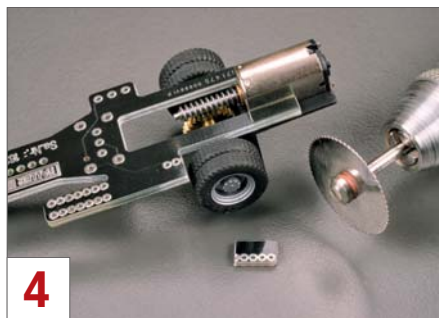
4 Für die gewünschte Platzierung des Antriebs müssen am Grundrahmen und am Halter störende Teile abgeschnitten werden.
