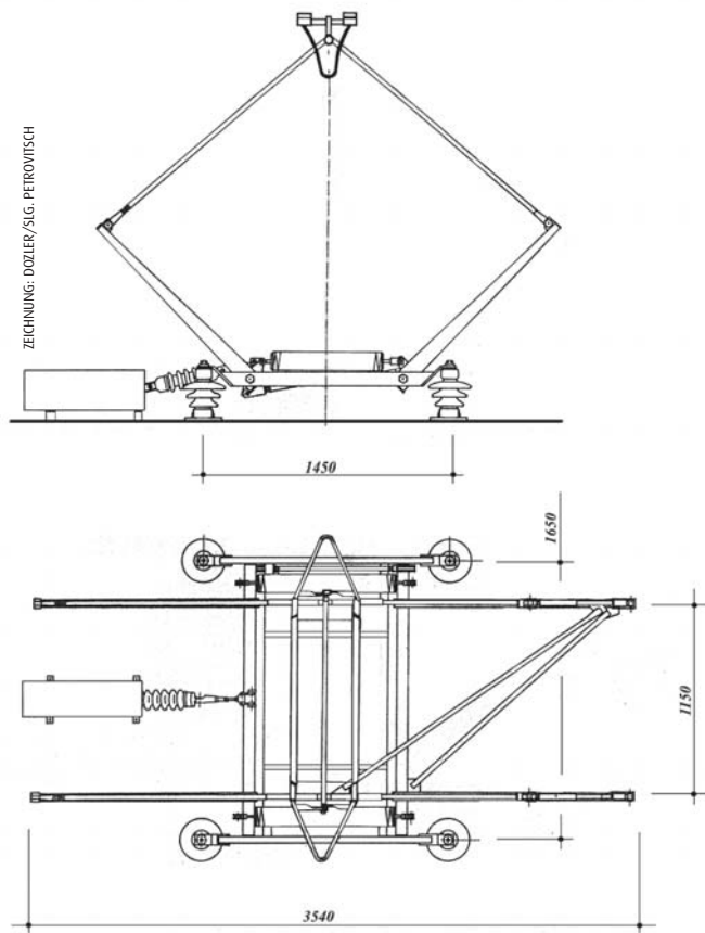
Zusammenstellungszeichnung des ab 1956 auf den DB-Einheits-E-Loks montierten Scherenstromabnehmers DBS 54.
