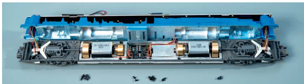
Nach dem Abnehmen des schweren blauen Gussteils mit der Inneneinrichtung fällt der Blick auf die beiden Motoren mit jeweils zwei Schwungmassen. Dazwischen liegt der Baustein zur Entstörung der Motoren.
