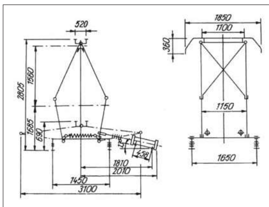
Die E 42 wurden, wie viele weitere DR-E-Loks, mit Stromabnehmern des Typs VS 18-25D ausgestattet.
