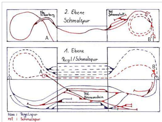
Die H0e-Strecke führt über eine Gleiswendel hinauf zu den Bergstationen, auf der unteren Ebene verläuft eine Durchgangsstrecke.
