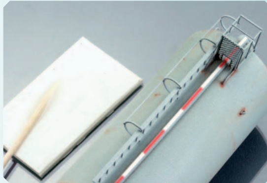
Der dünne Blechstreifen wird am besten mit wenig Uhu-Plus auf der nach oben laufenden Rohrleitung des Tanks fixiert.
