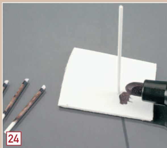
24 Die hölzernen Begrenzungsposten entstehen aus 1,2 mm dickem Evergreen-Kunststoff-Rundprofil.
