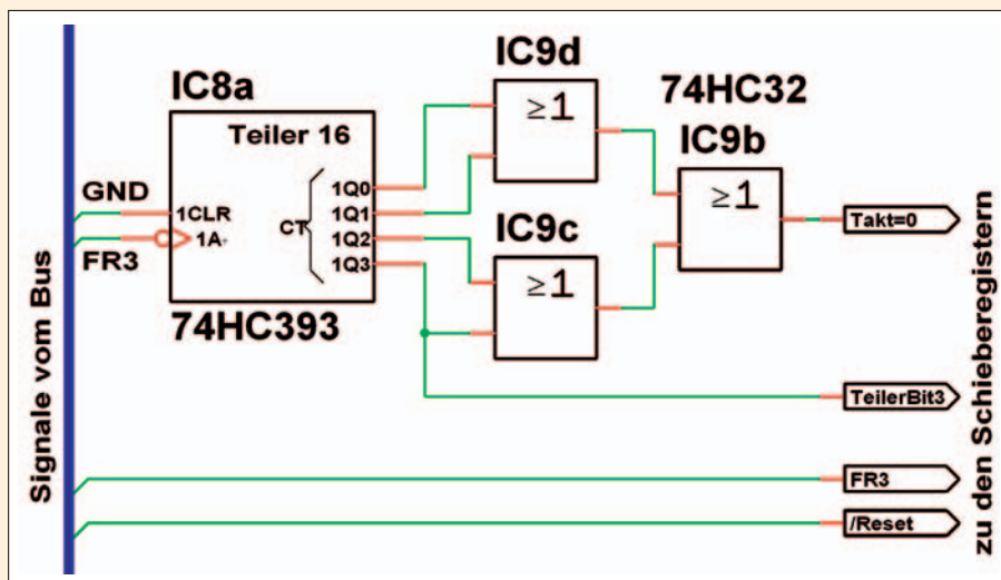
Takt-Erzeugung: Zur Steuerung der Schieberegister werden Signale vom Bus abgegriffen.
