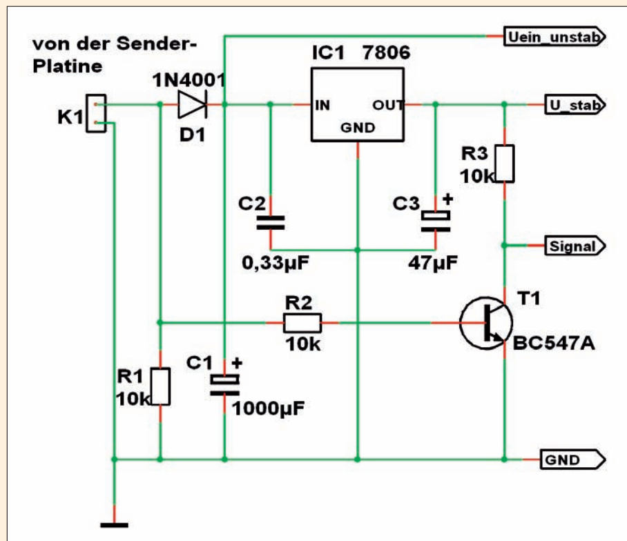
Stromversorgung: Die von der Steuerung kommende Ader führt die rhythmisierte Spannung.
