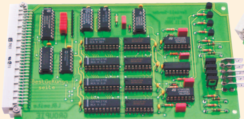
Der erste Prototyp der Senderplatine: Gut zu erkennen sind die Flachstecker, die vor allem in der Kfz-Elektrik Verwendung finden.
