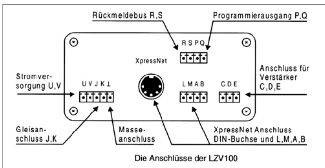
An der Rückseite der LZV 100 finden sich die diversen Anschluss-Buchsen.
