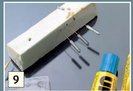
Die transparenten Abdeckungen der Leuchtmittel stellt man mit Uhu-Plus-Kleber dar.
