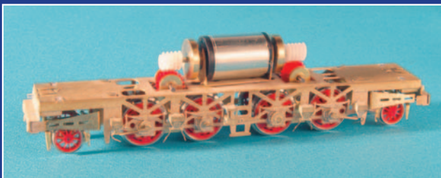
Filigran: Rothes TT-E17 erhält einen maßstäblich breiten Rahmen.
