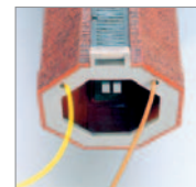
Die Litzen werden durch in die Standfläche gebohrte Löcher sauber in die Bodenplatte geführt und dort an die Stromversorgung angeschlossen.
