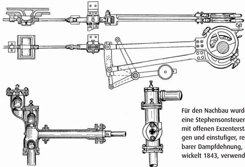
Zeichnung: Aus Schienenfahrzeuge 2/1989
