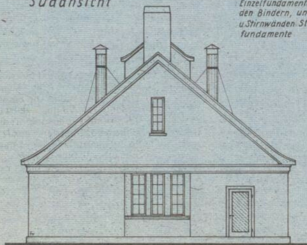
Südansicht
