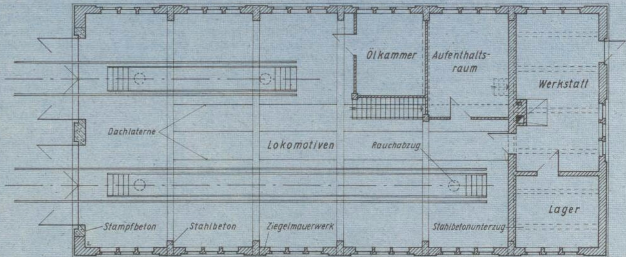
Grundriß
