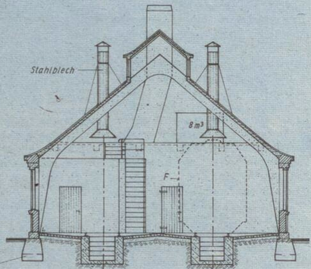
Querschnitt
