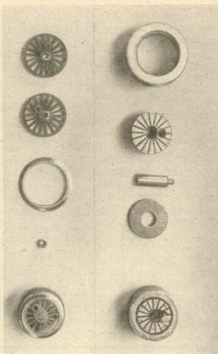
Linke Reihe: zwei Radsternrohlinge, Radreifen ( \varnothing 20 mm), Radbuchse, komplette Kuppelachse ( \varnothing 16,5 mm).
