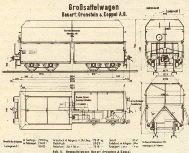
Abb. 11. Grossattelwagen Napert Orenstein &amp; Koppel
