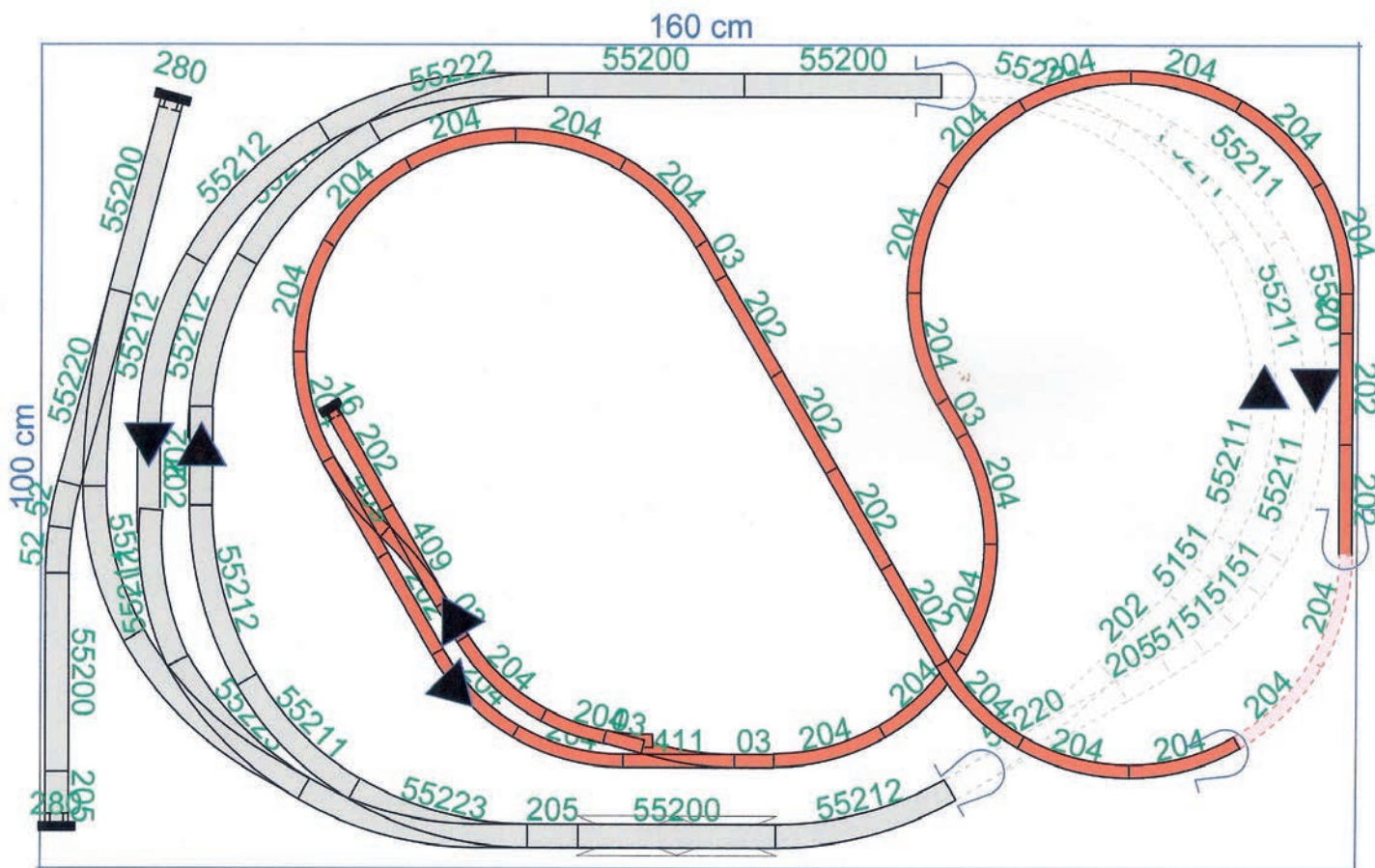
Der Gleisplan in der Originalausführung für Piko-A-Gleis und H0e-Gleis von Roco.
