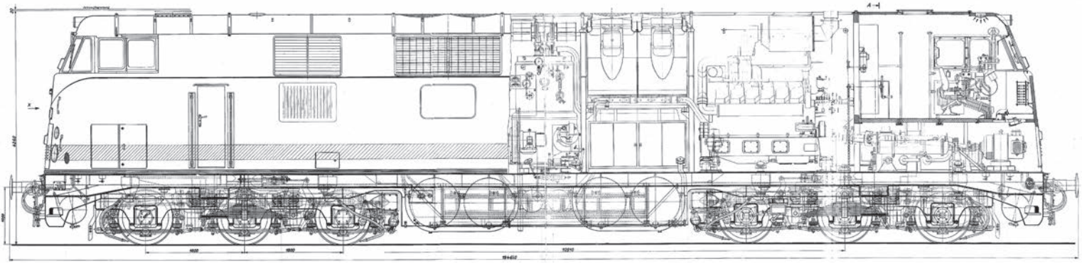
Längsschnitte der V 180.0 (links) und V 180.1 sowie Datenblatt der V 180 C'. ABB.: SLG. MÜLLER (2), SLG. KOSCHINSKI (3)
