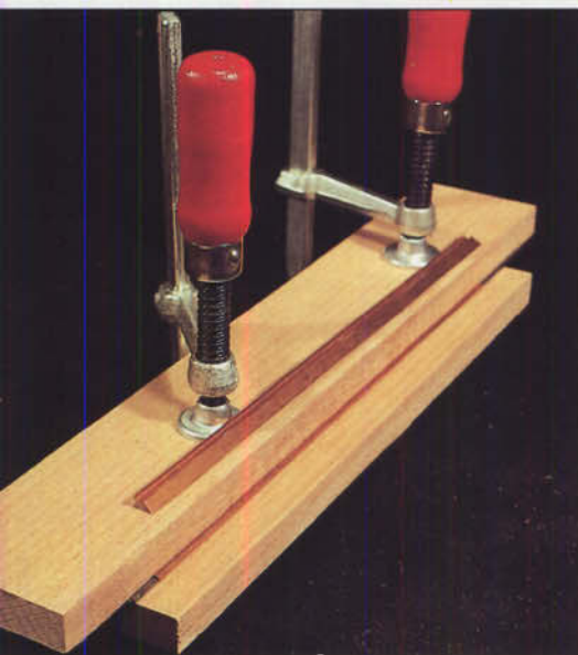
Bilder 25 und (unten) 26: Mit Hilfe der hier gezeigten Vorrichtung wurde auch die Dachrinne für das Lagerhaus aus Kupferfolie selbst hergestellt. Zwischen zwei Hölzern fixiert, wird die Folie über einen ca. 2 bis 3 mm starken Draht zu einer Rinne gebogen. Auf dem oberen Holz liegt eine schon fertige Rinne.
