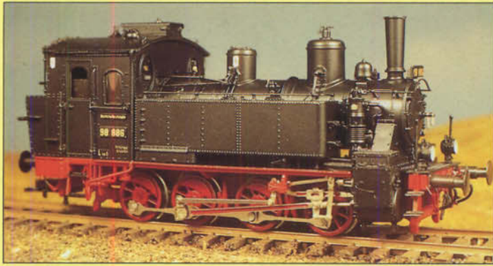
Bild 13: Auf dem H0-Fahrwerk von Fleischmann gestaltete die Berliner Firma Reitz eine wunderschöne GtL 4/4 als 98 886 der DRG.
