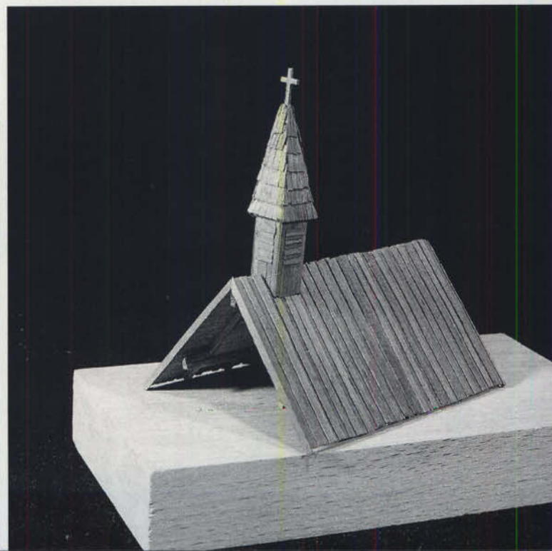
Bild 32: Selbst die Unterseite des abnehmbaren Kapellendachs ist vorbildgerecht detailliert. Das Gebälk wurde in allen Einzelheiten durchgebildet.
