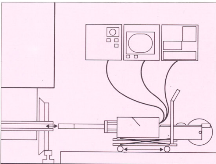
Manipulator mit der Steuer- und Auswerteeinheit. Hier werden die Prüfergebnisse ausgewertet und Werkstofffehler auf einem Monitor dargestellt bzw. per Videorecorder gespeichert.
