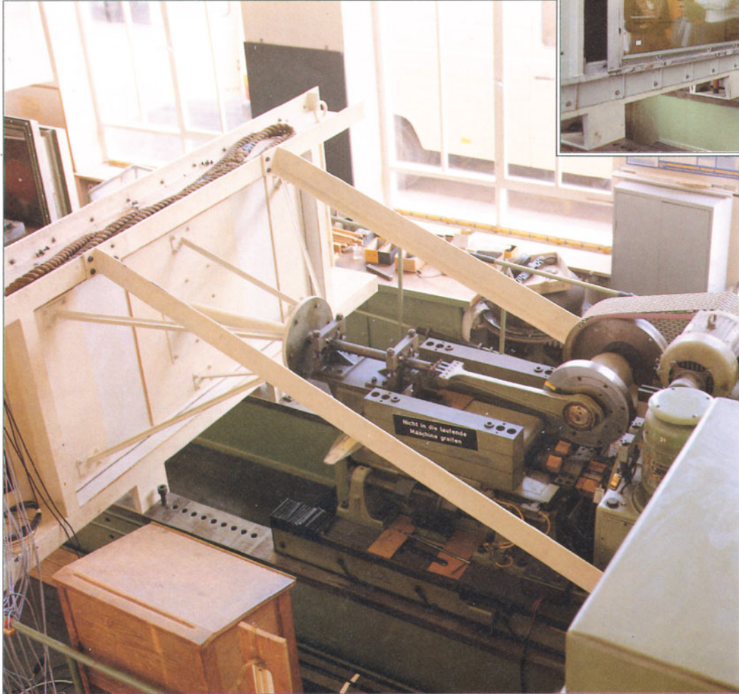
Bild 4: Wie mit einer überdimensionalen Luftpumpe wird die Luft mit definiertem Druck an die Scheibe gepreßt.
