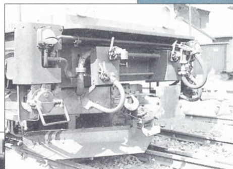
Bild 2: Die Mittelpuffer-Schraubenkuppelung dient dem Kuppeln mit Personenwagen, die Trichter-Kuppelung darunter ist für die Kuppelstangen der Rollfahrzeuge bestimmt.
