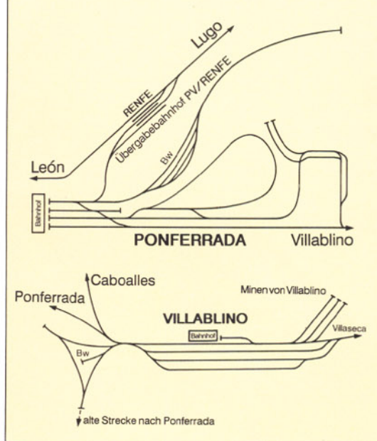
Bild 8: Schematische Darstellung der Gleisanlagen in Ponferrada und Villablino (nach einer Vorlage von Thierry Leleu). Zeichnung: G. Voigt
