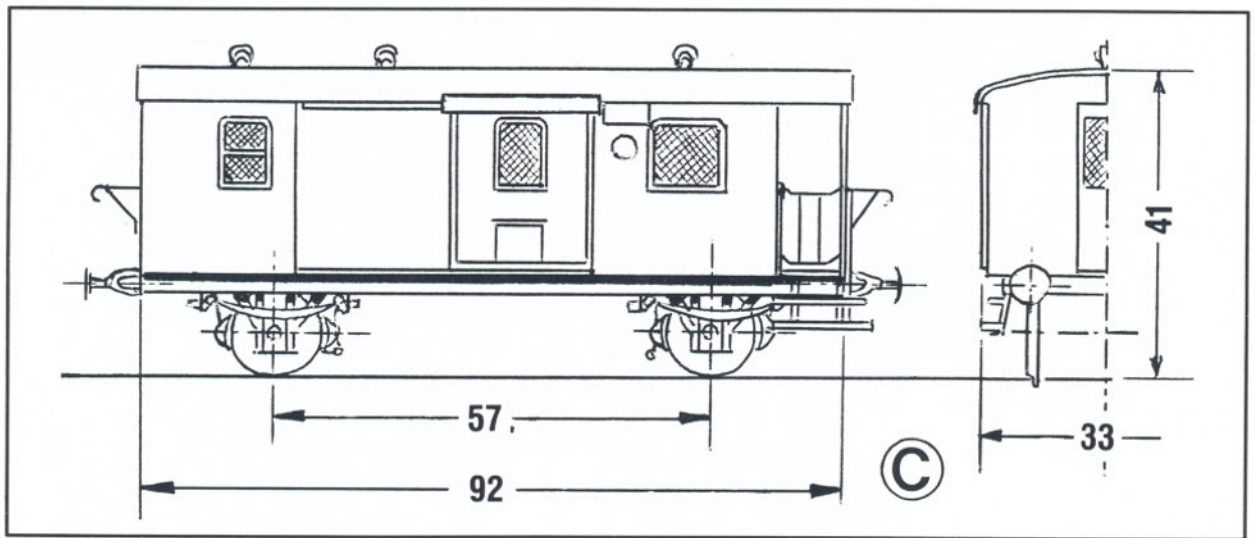
Bild 10: ... und zum Selbstbau des Wagenkastens. Zeichnung: Dr. Hufnagel
