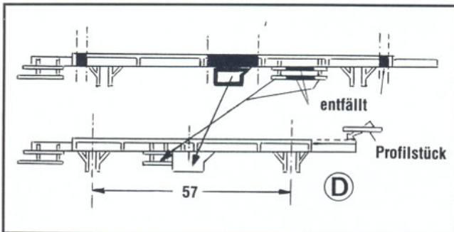
Bild 9: Anleitung zum Zuschchnitt des Fahrgestells ... Zeichnung: Dr. Hufnagel
