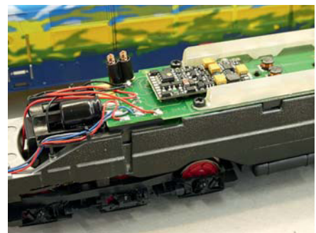
Das elektrische Potential des Lok-Mittelschleifers wird über stromleitende Kupplungen an die Wagen weitergereicht.
