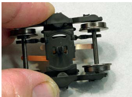
Die Drehgestelle lassen sich einfach ausklipsen, um die Radsatzmaße zu prüfen. Man beachte die Lage der Isolierbuchsen!
