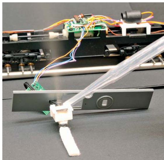
Nach Lösen von zwei Schrauben kann er abgehoben werden. Nun sind Decoder und Schnittstellenplatine zugänglich. Der schwarze „Knubbel“ links ist ein Kondensator, der die SUSI-Spannung puffert.
