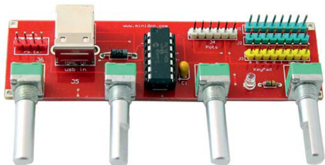
Links hinten in Rot der UART-Anschluss, daneben USB. Ganz rechts der Keypad-Anschluss, in Türkis für normale „flat“-Ansteuerung, in Gelb für Telefon-Tastaturen. In Weiß daneben eine weitere Möglichkeit Potentiometer anzuschließen.
