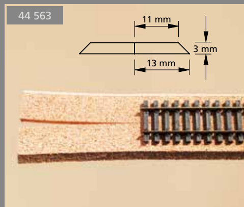
44 563 Korkgleisbettung für Schienen Cork track underlay for track
