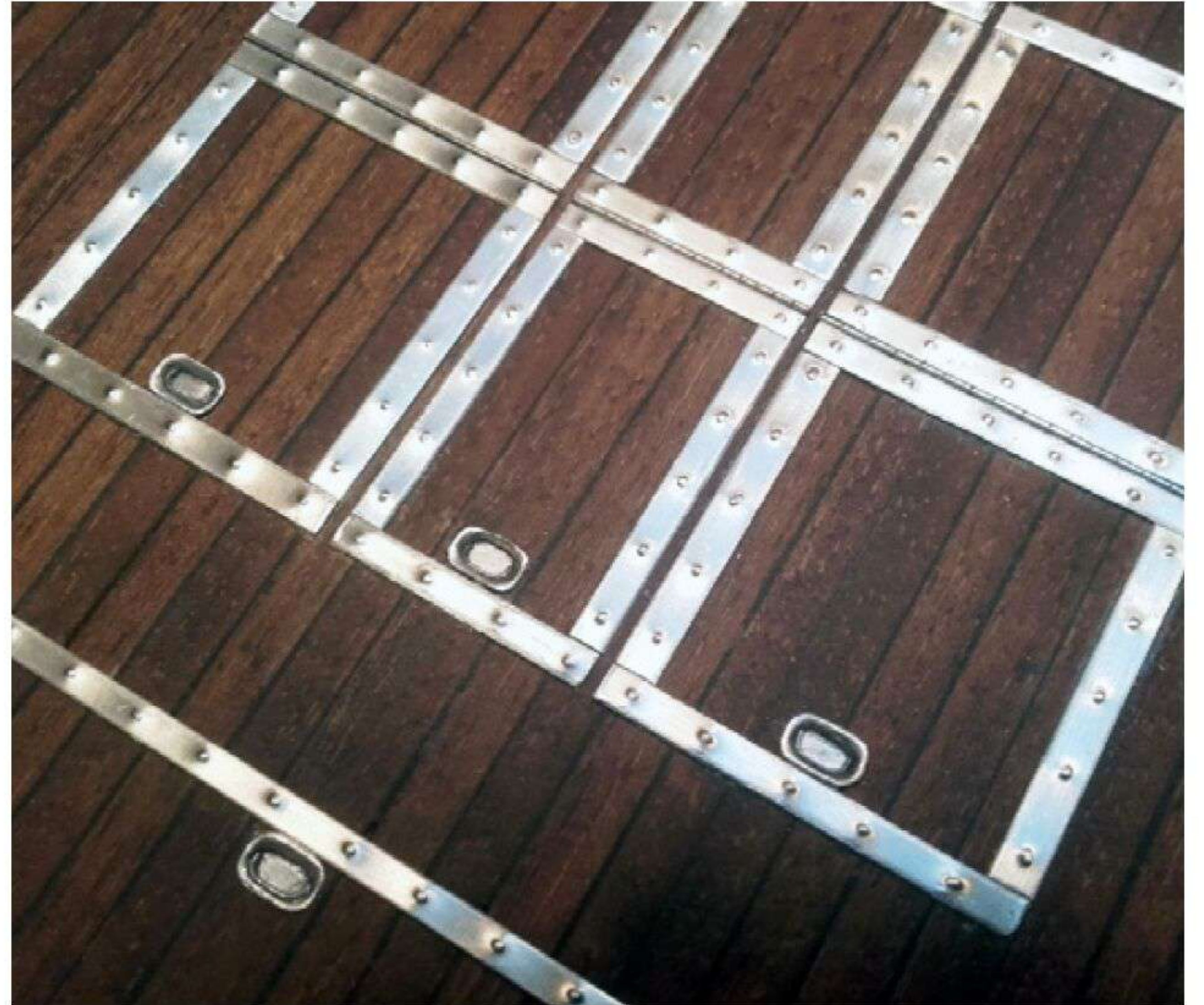
Die Lukenrahmen bestehen aus dünnem Alublech und wurden mit Nieten und Scharnieren versehen
