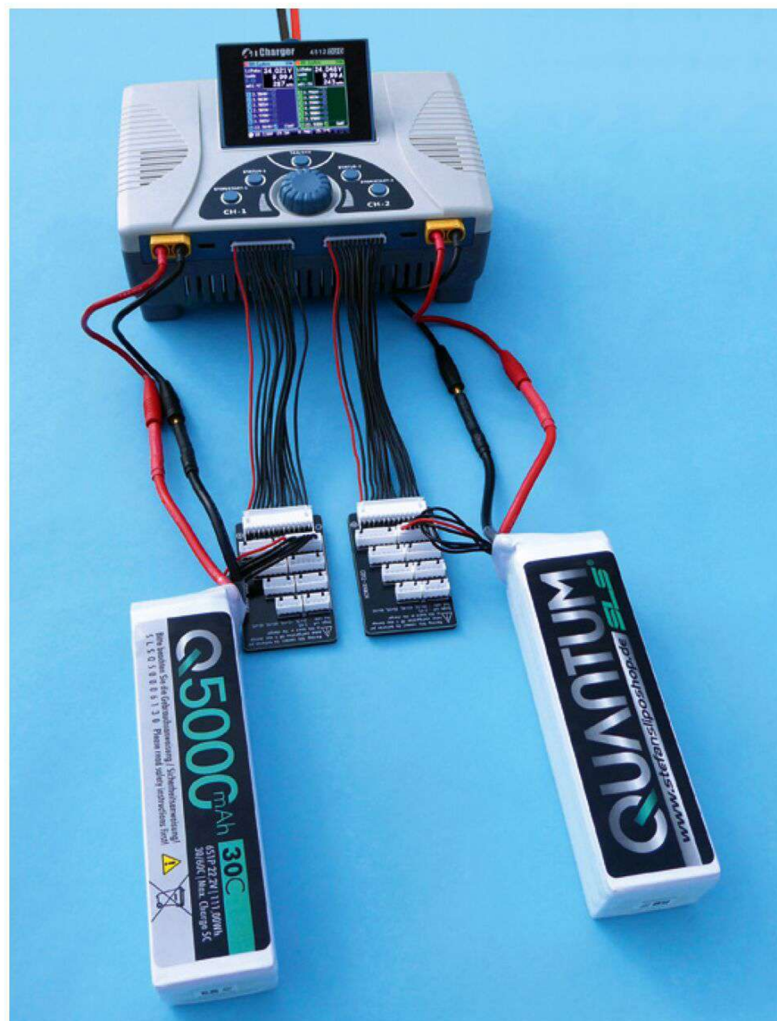
Ladevorgang von zwei LiPo-Akkus mit je sechs Zellen
