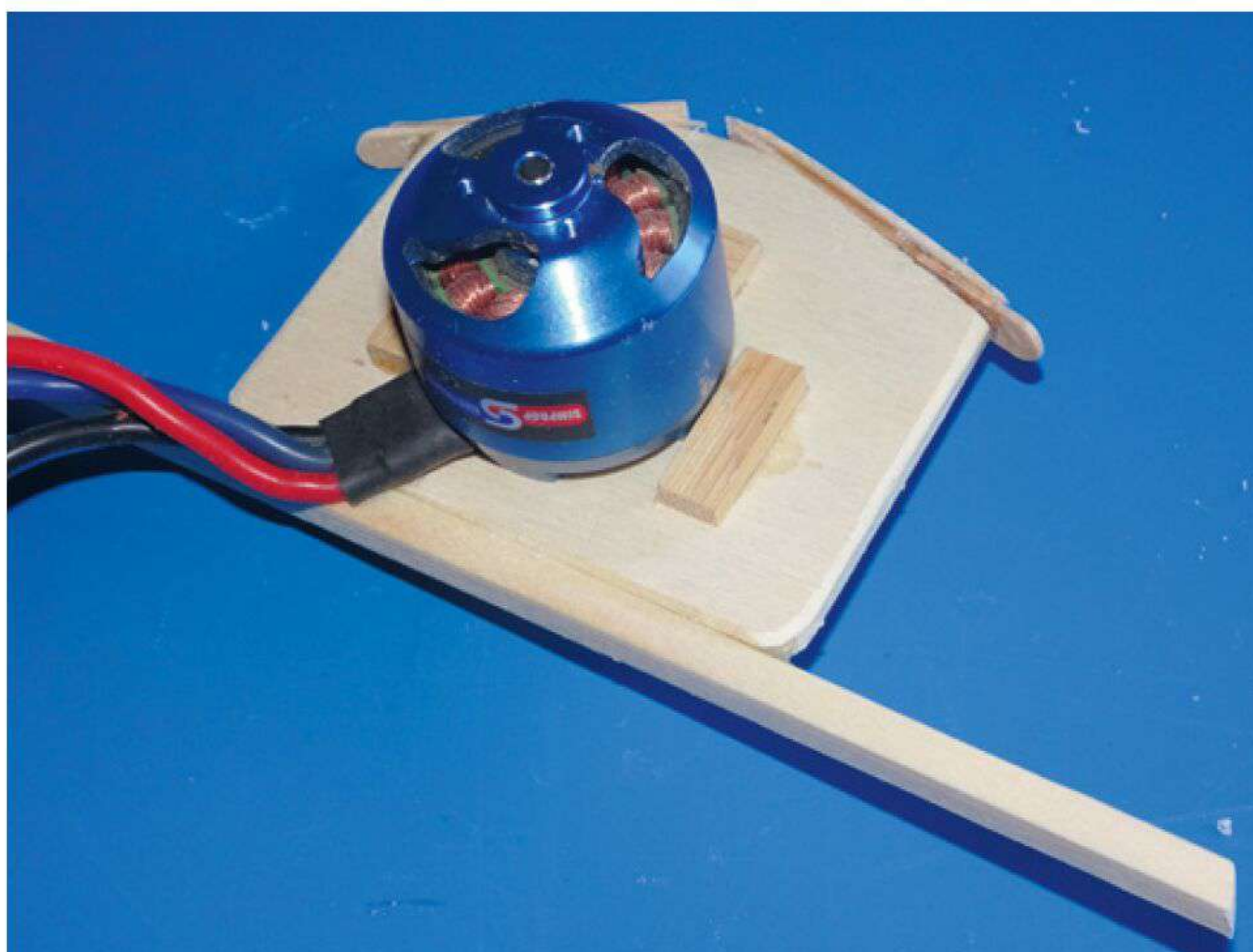
Mit der oberen Leiste stützt sich der Motorspant später an den Rumpfseiten ab
