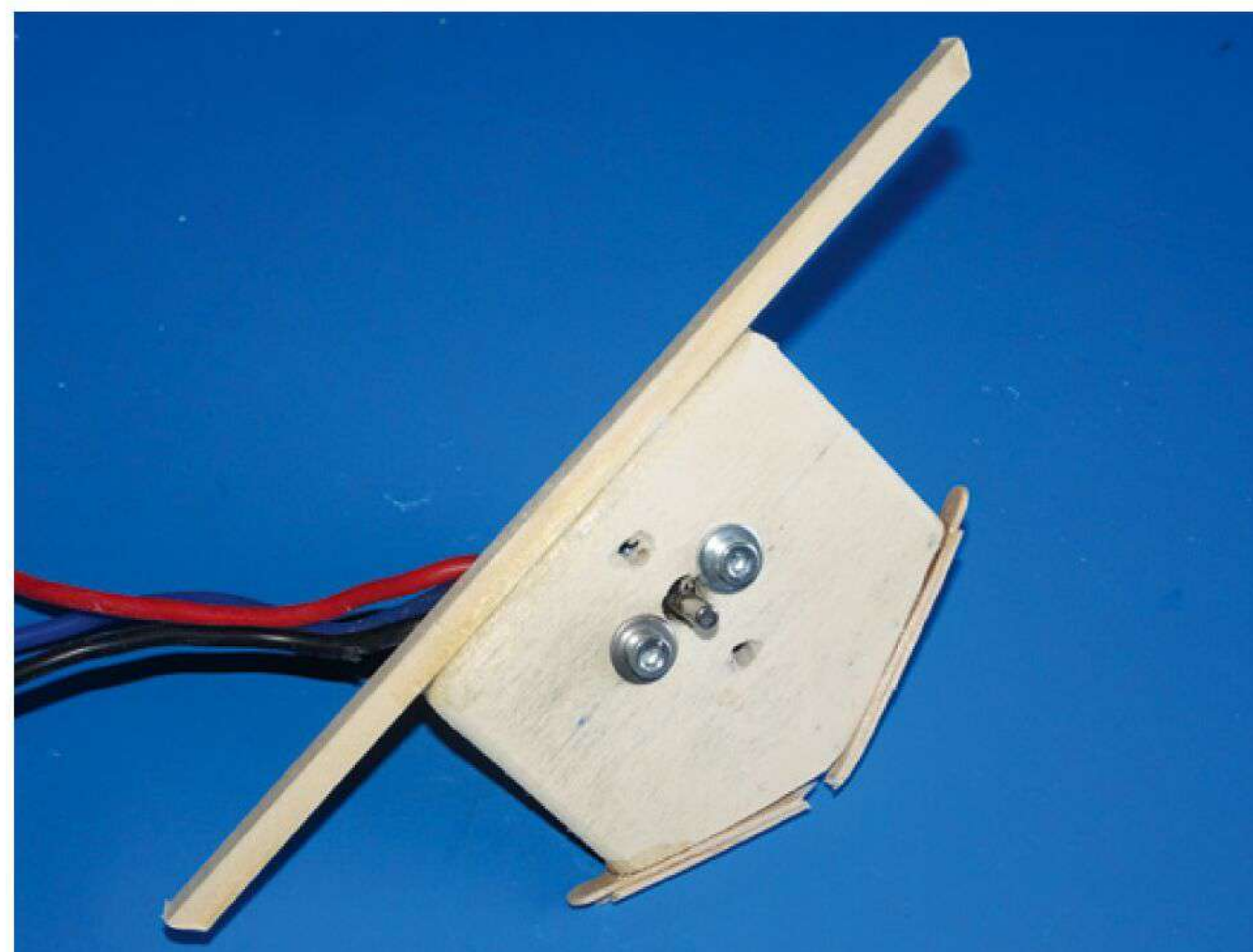
Die Motoren werden mit Inbusschrauben angeschraubt, da sich diese später in dem engen Rumpf besser lösen lassen, falls nötig
