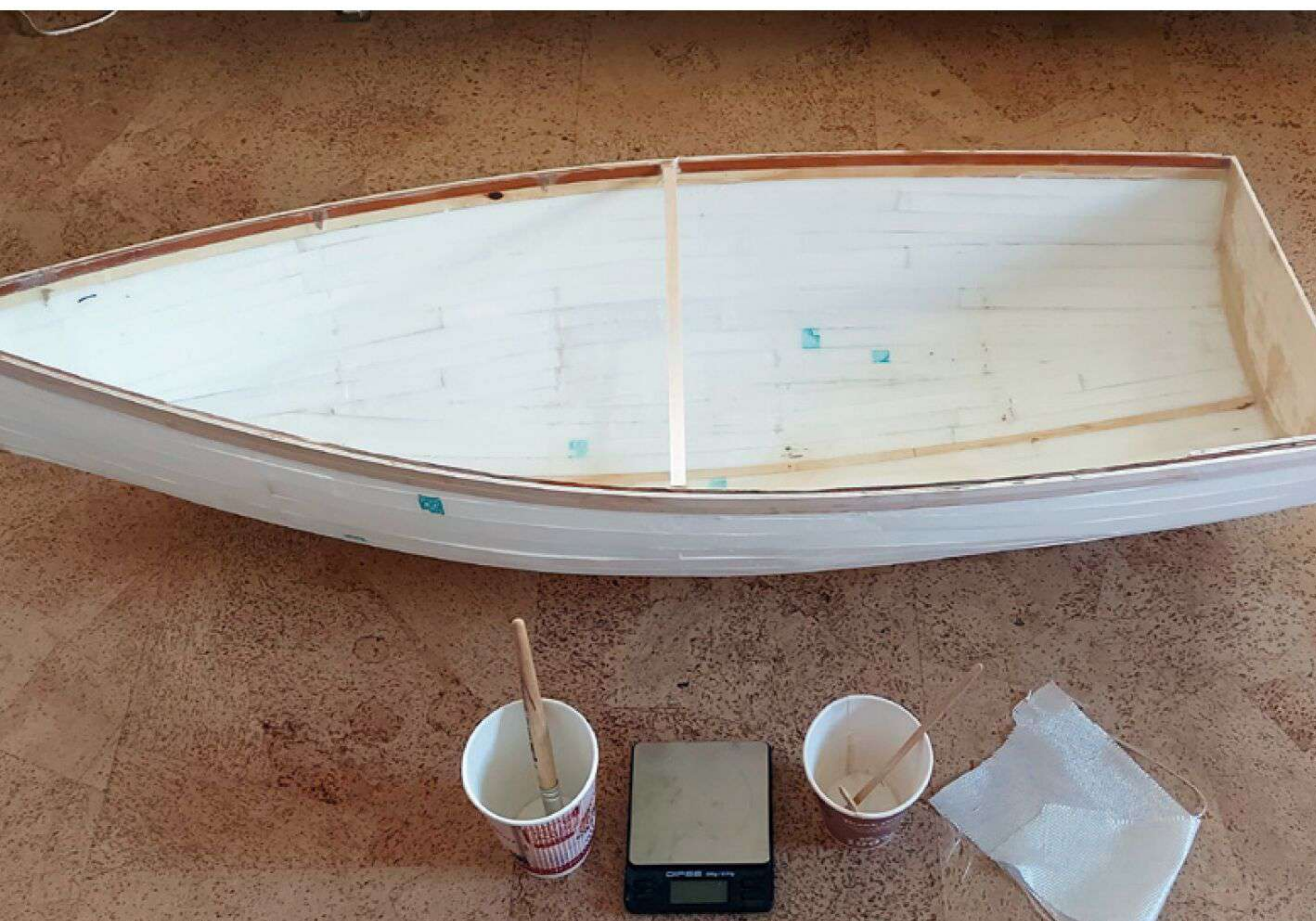
Zur Stabilisierung wurde der Rumpf innen mit Glasgewebe laminiert
