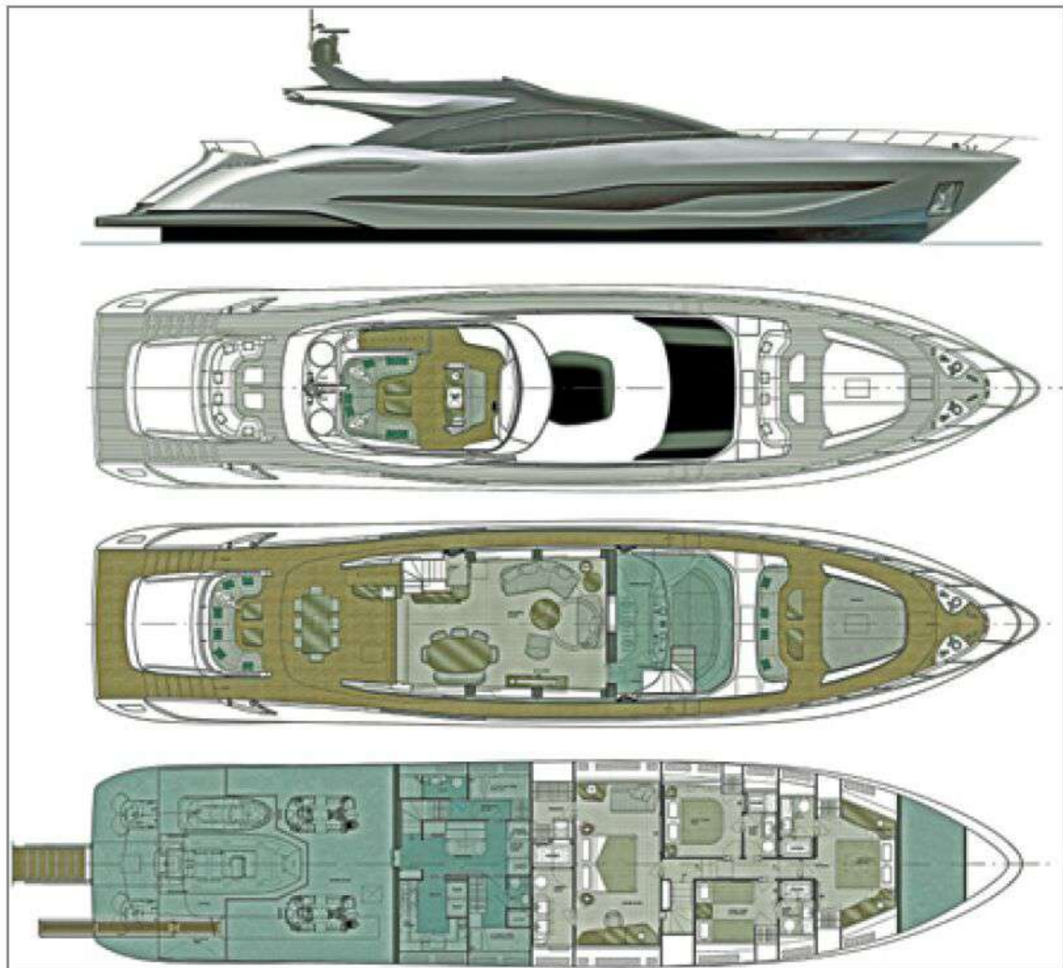
Seiten- und Decksansichten der Mangusta 104 REV
