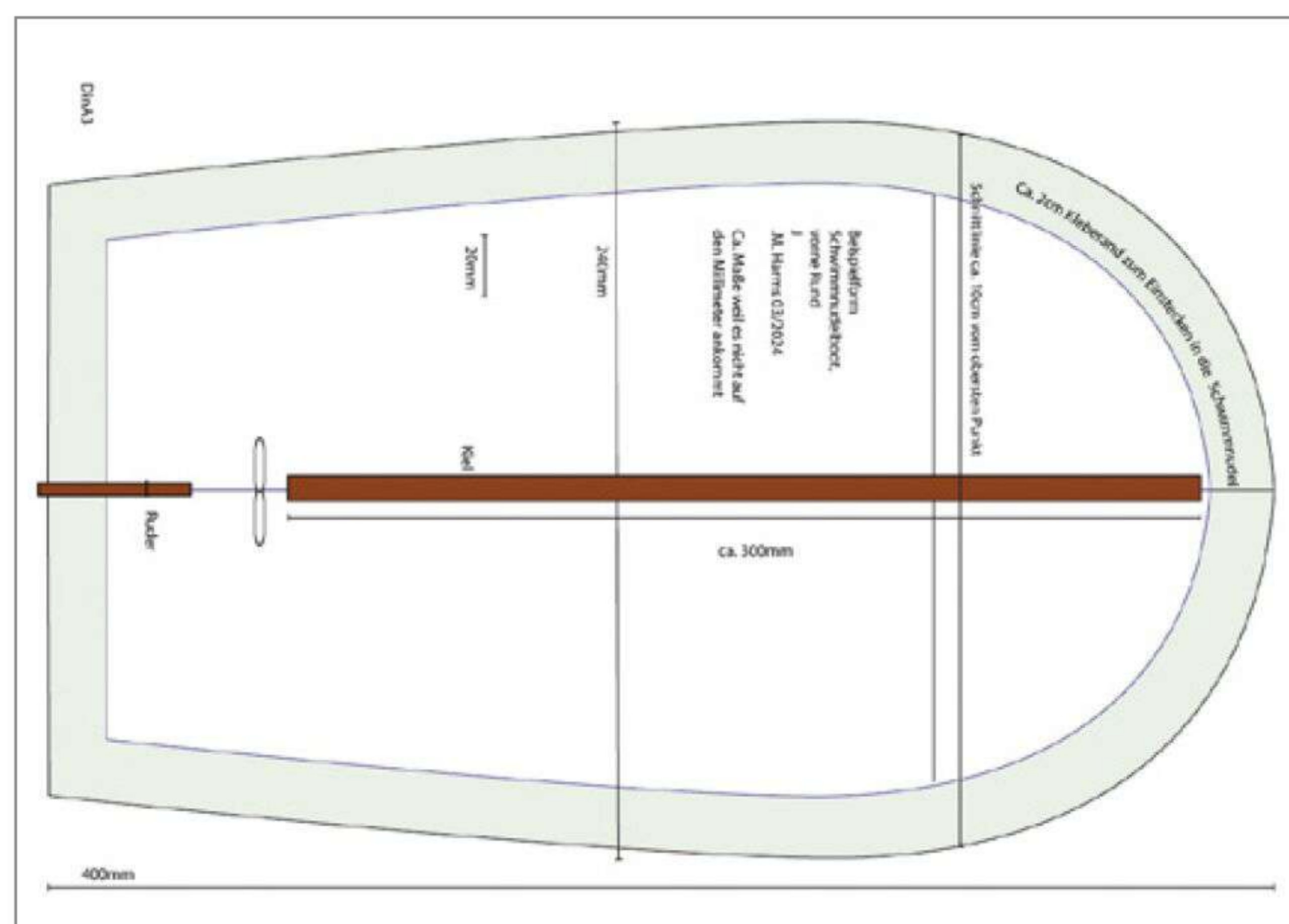
Dieser Bauplan ist auf www.schiffsmodell-magazin.de kostenlos verfügbar
