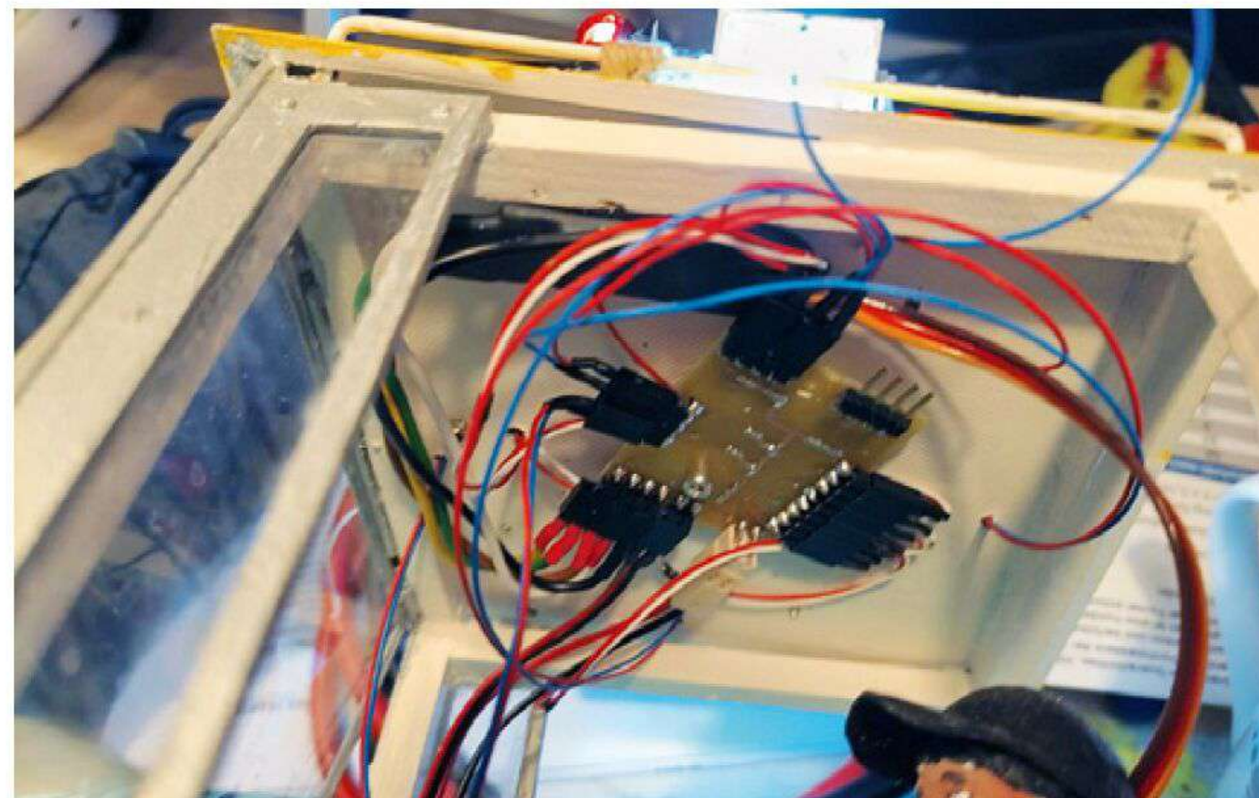
Die Beleuchtungsverteilung ist unter dem Kabinendach angebracht
