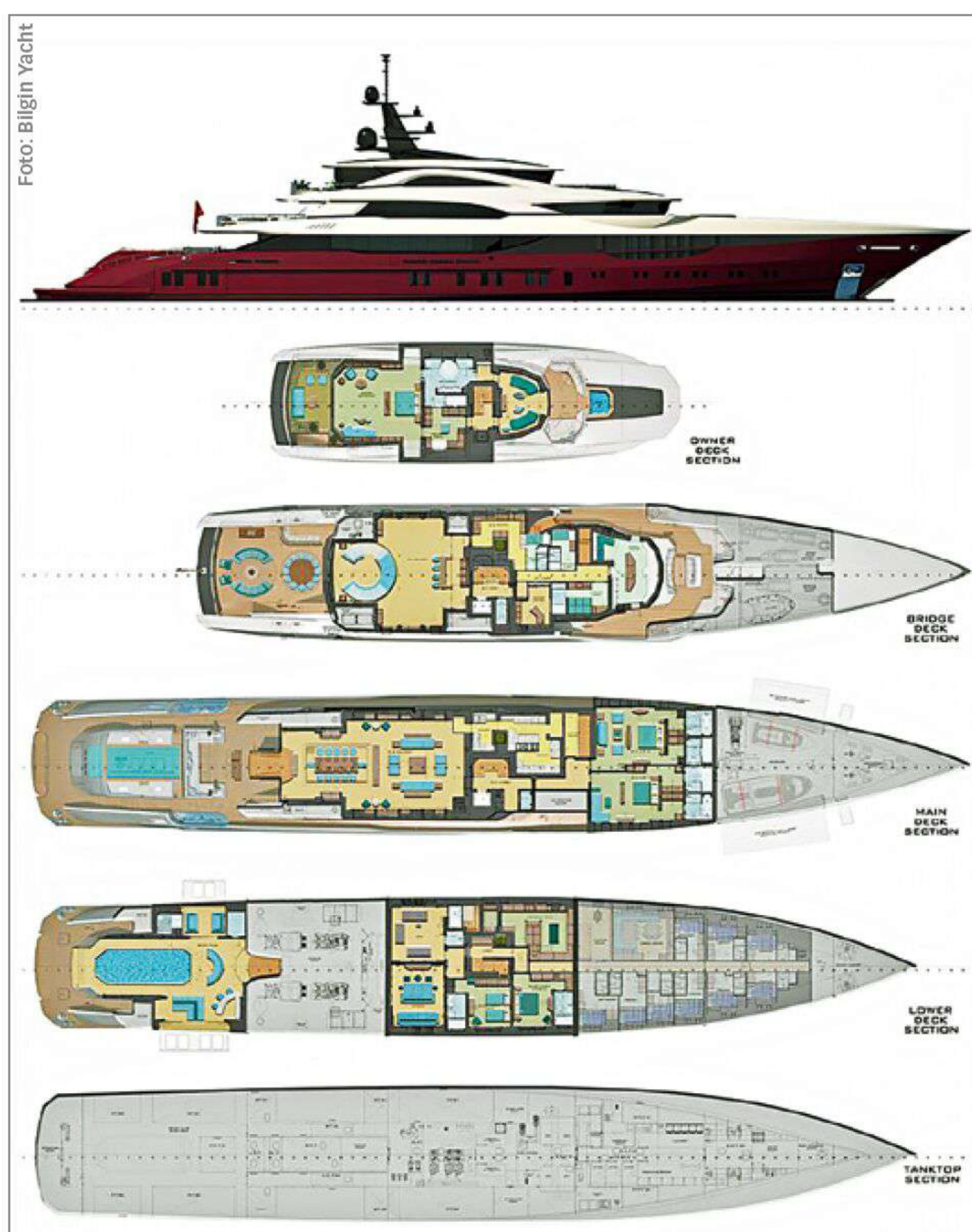
Seiten- und Decksansichten der Bilgin-Yacht LEONA
