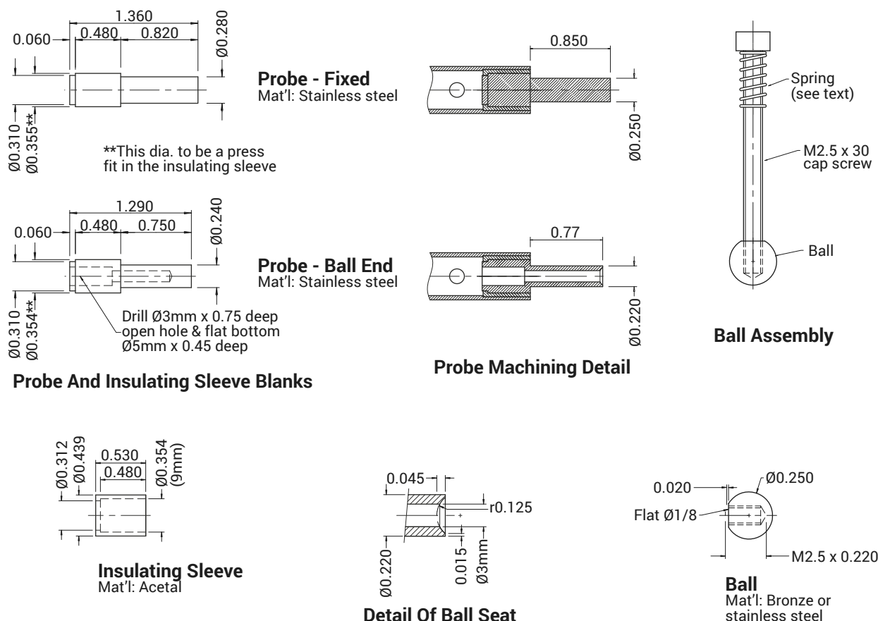
Fig.6 Probes
