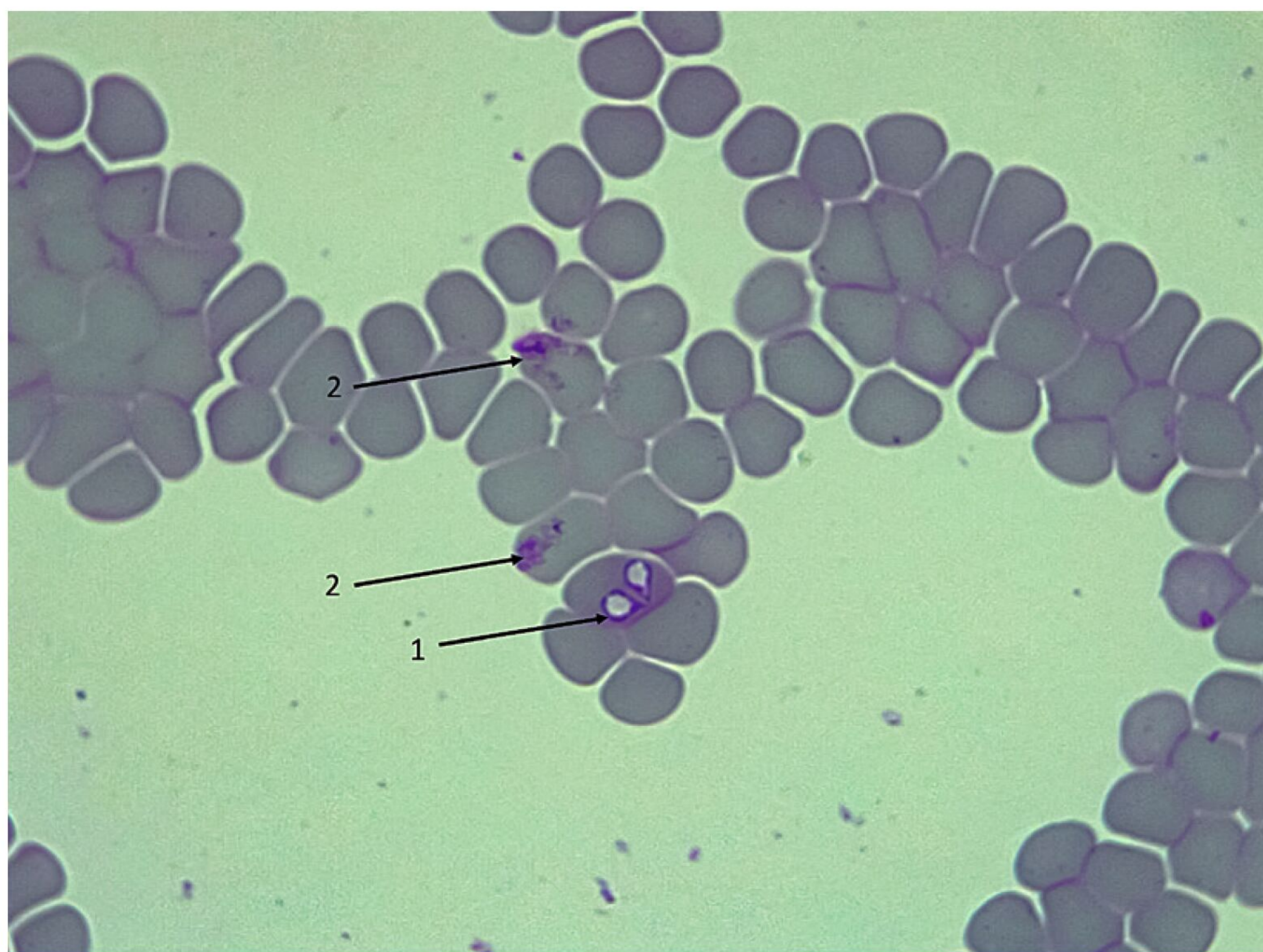
Unter dem Mikroskop: Babesia in Hunde-Erythrozyten
