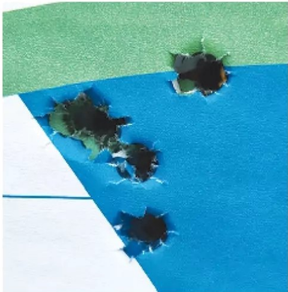
Corbon 62-grain T-DPX.
