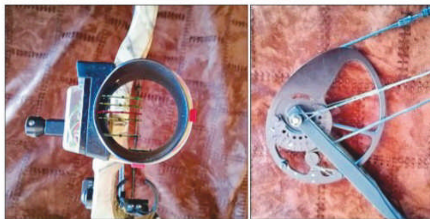
'n Visier met verskeie penne ( pins ) aan die voorkant van 'n boog.
