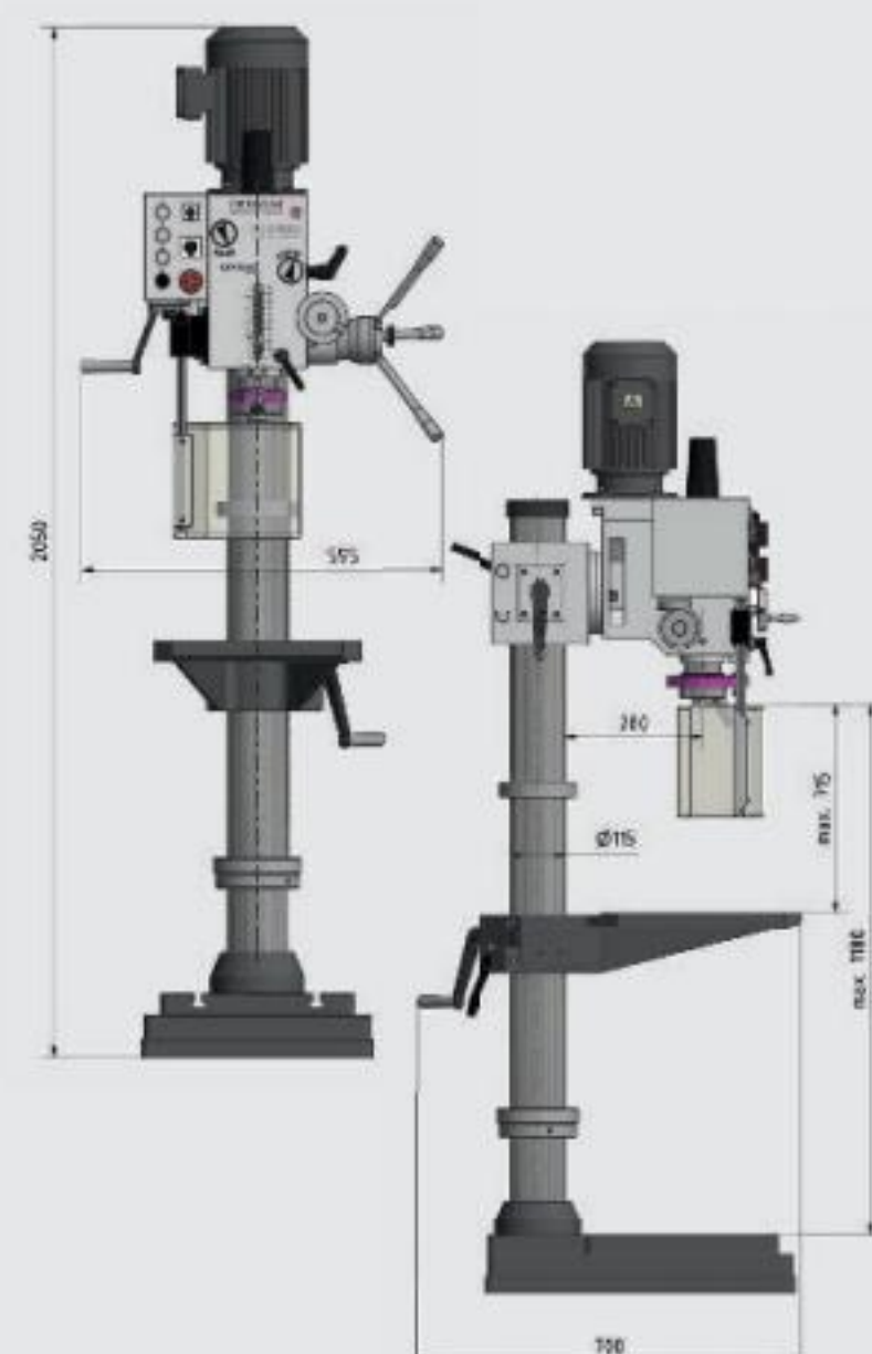
Dimensions DH 40G
