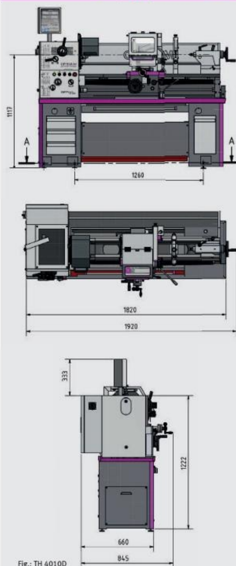
Fig.: TH 4010D
