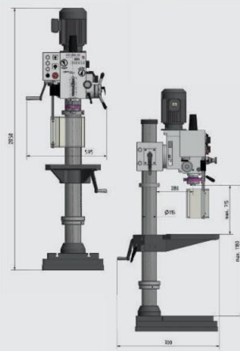
Dimensions DH 40GP
