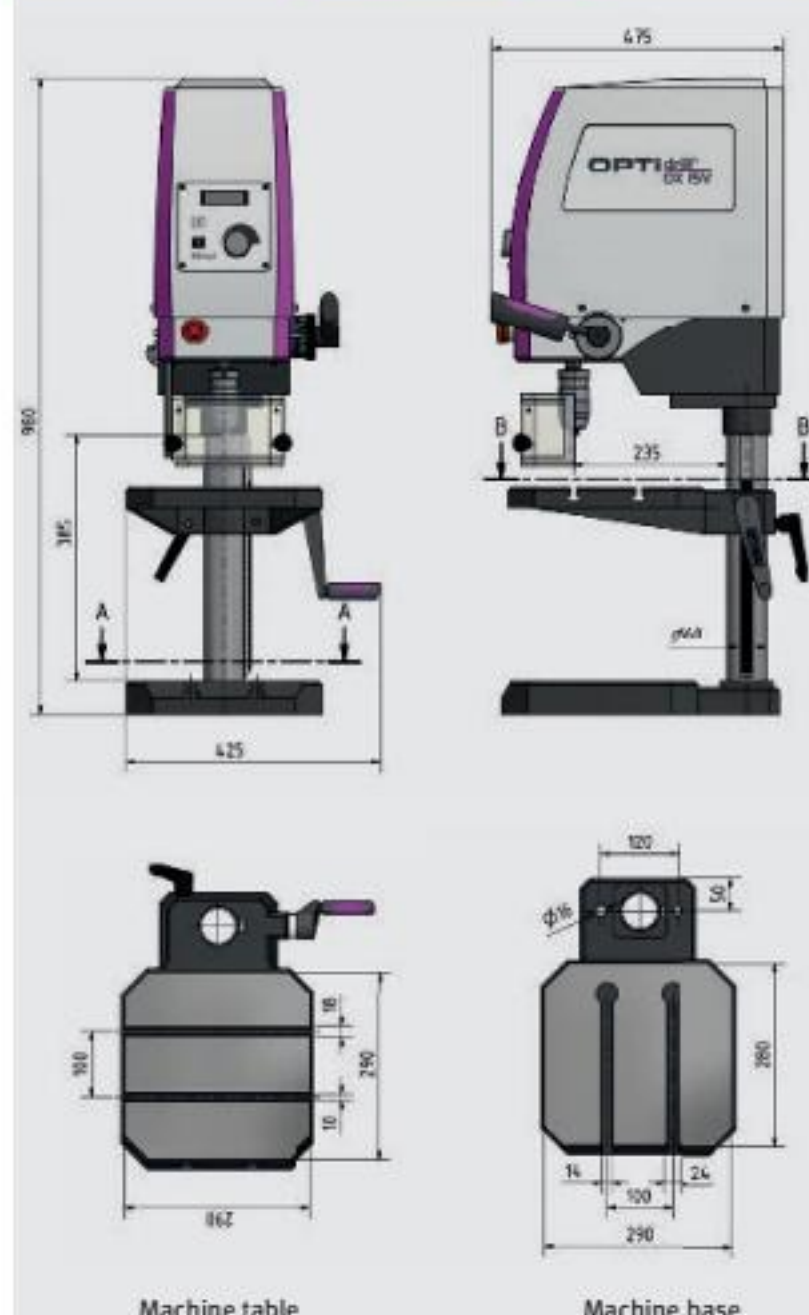
Dimensions DX 15V
