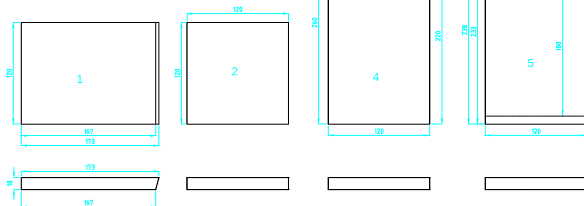
Vogelhuisje voor een pimpelmees
