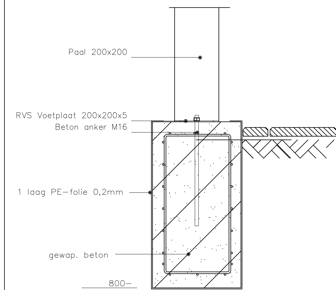
DETAIL FUNDERING ONDER PAAL
