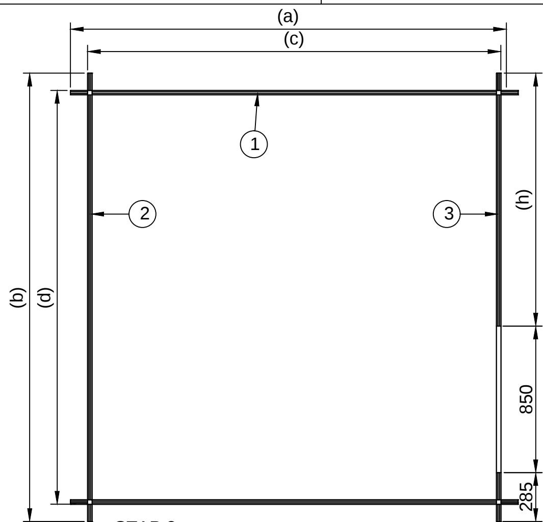
STAP 2: 1e laag blokhutplanken aanbrengen
