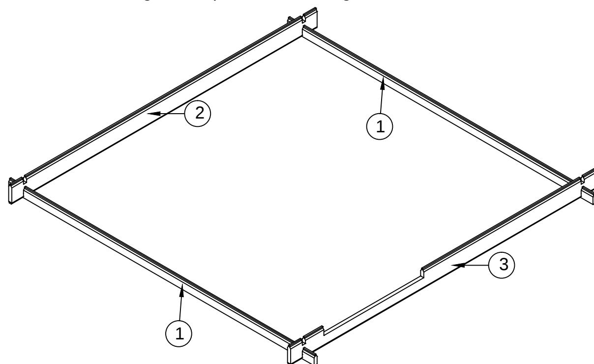
STAP 2: 1e laag blokhutplanken aanbrengen
