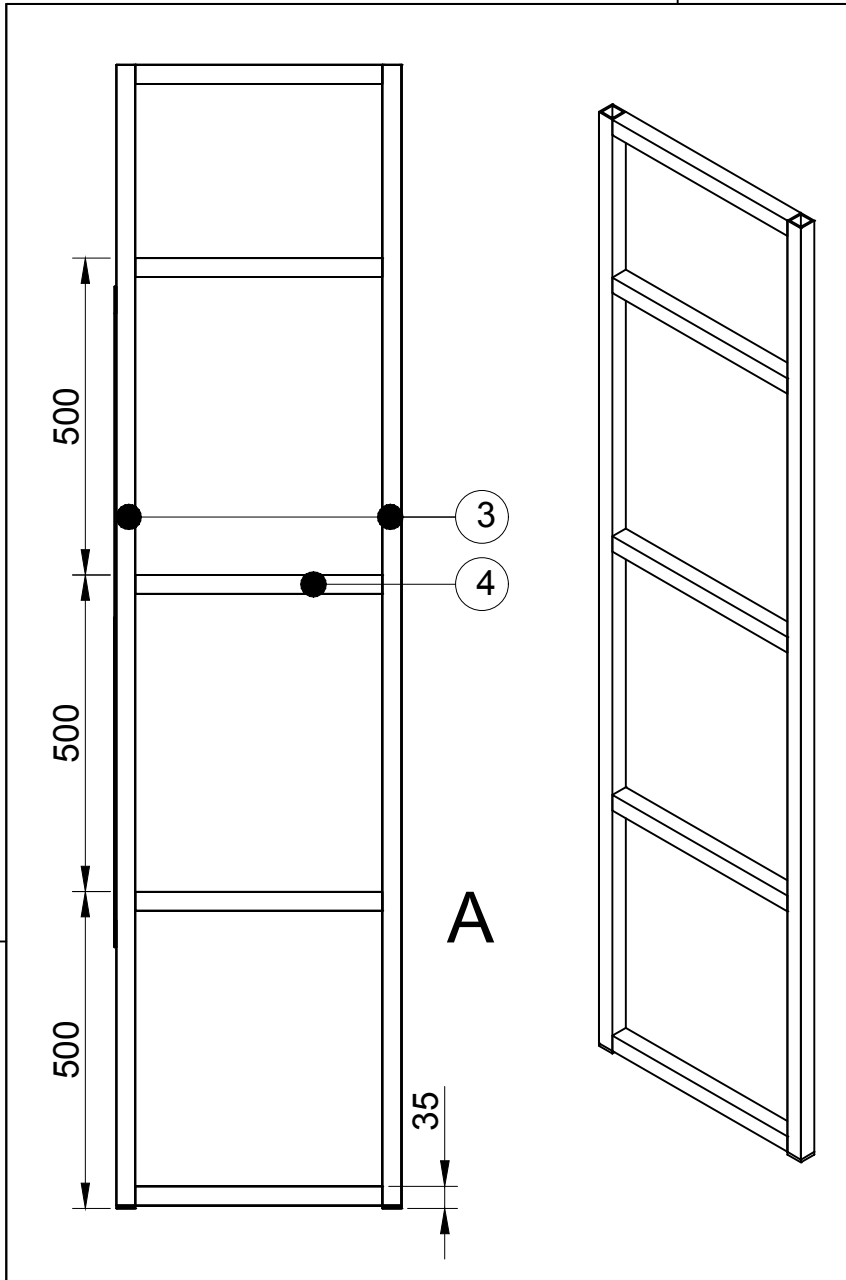
Staal lassen
