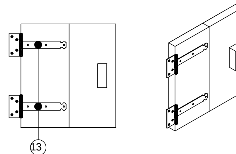
Hengens aanbrengen aan deurtje
