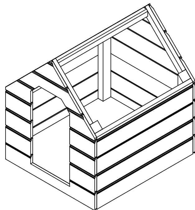
Voorwand vastschroeven
