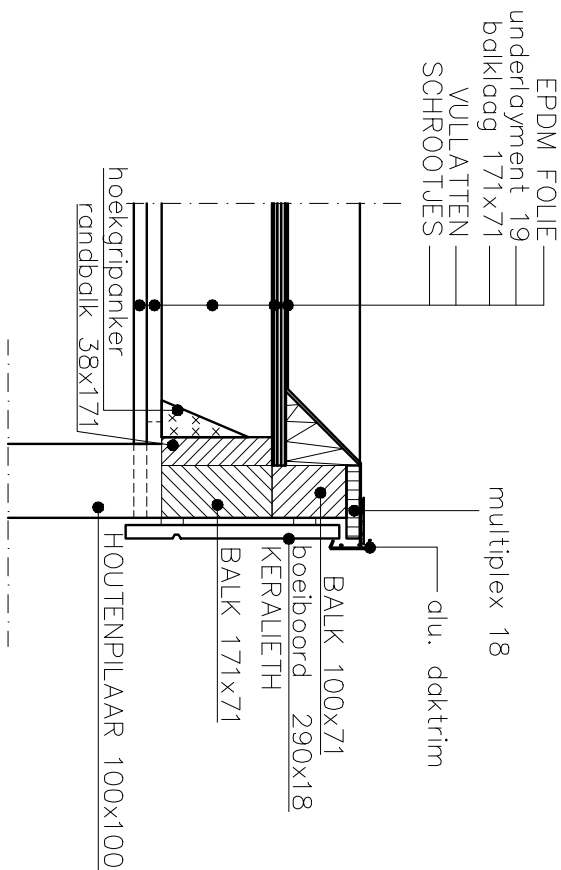
PRINCIPE DETAIL PLATDAK Schaal 1:10
