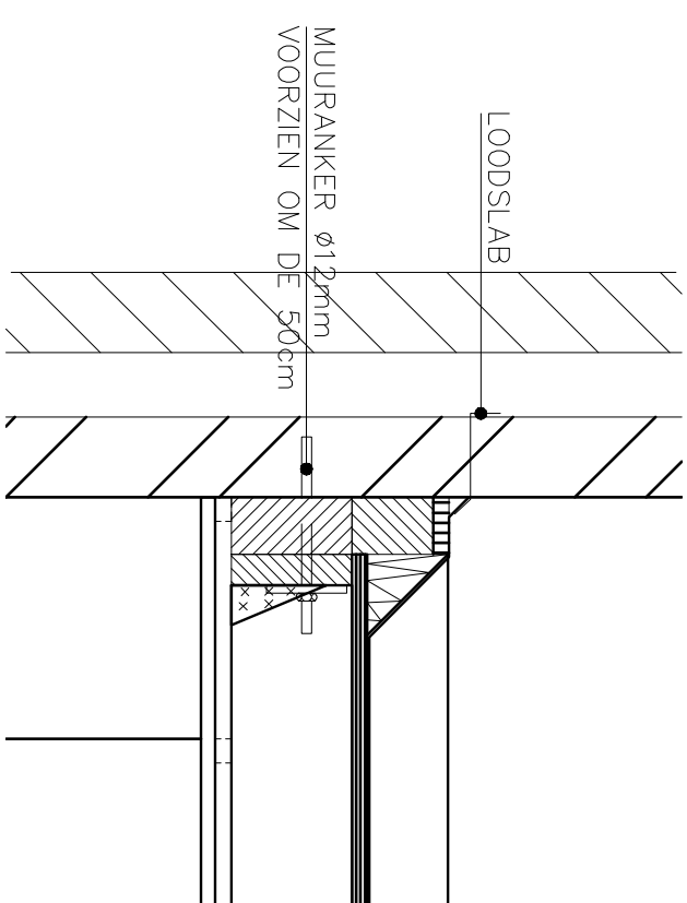
PRINCIPE DETAIL AANSLUITING PLATDAK OP BESTAANDE WONING Schaal 1:10
