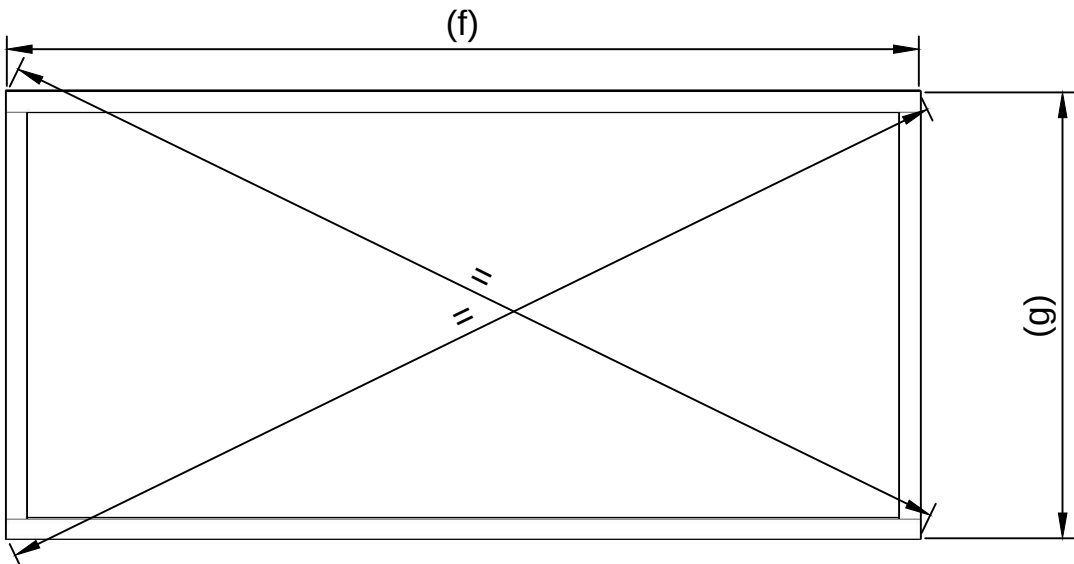
Frame overhoeks meten lengtes moeten gelijk zijn
