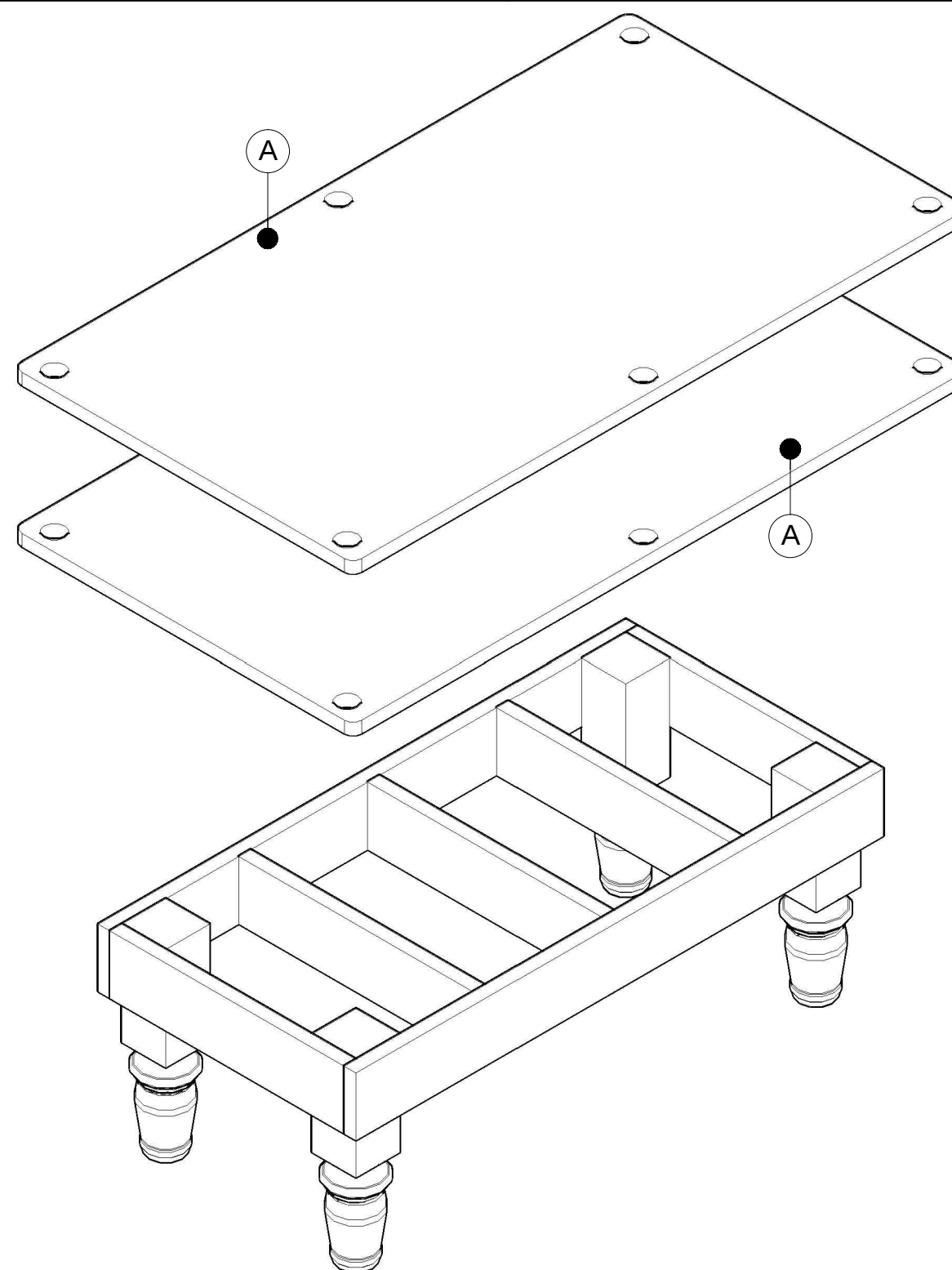
1e blad aanbrengen en vastschroeven 2e blad vastlijmen op eerste blad
