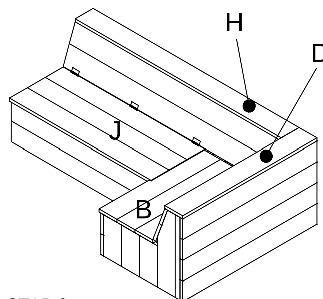
STAP 6 1. Scharnieren voorzien 2. ITEM J 3. ITEM B
