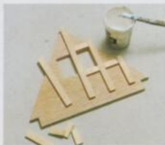
De decoratieve vakwerkgevel bestaat uit 15 x 3 mm dikke latjes.
