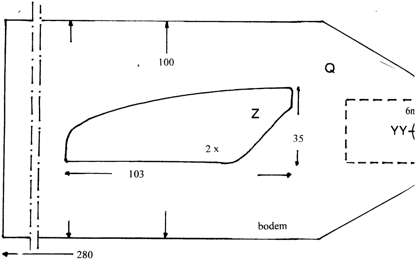
zijaanzicht
