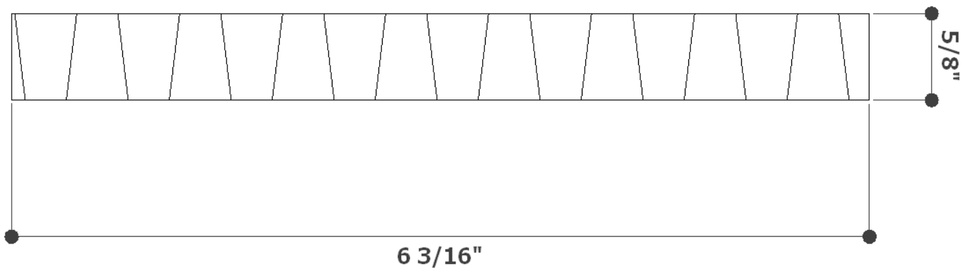
Pièce aa (arrière de tiroir) vue de côté
