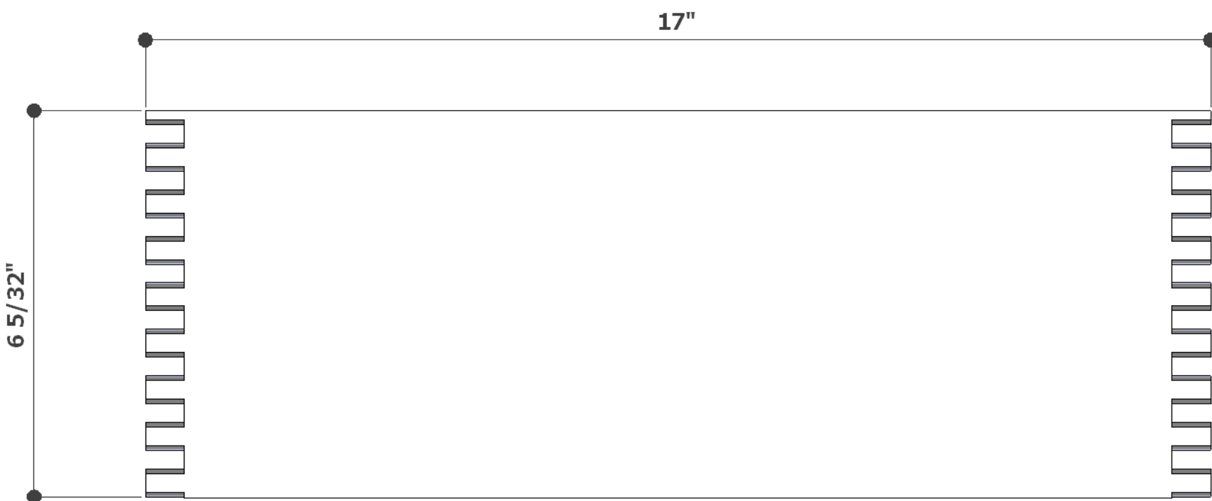
Pièce aa (arrière de tiroir) vue de face
