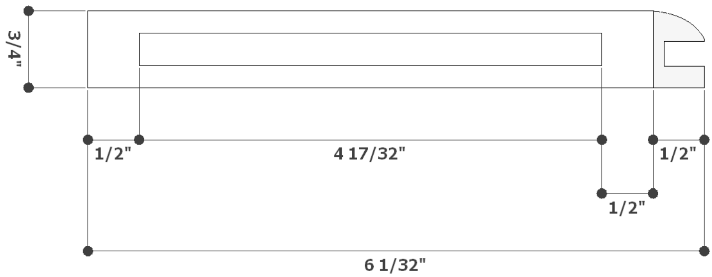
Pièce g vue du devant
