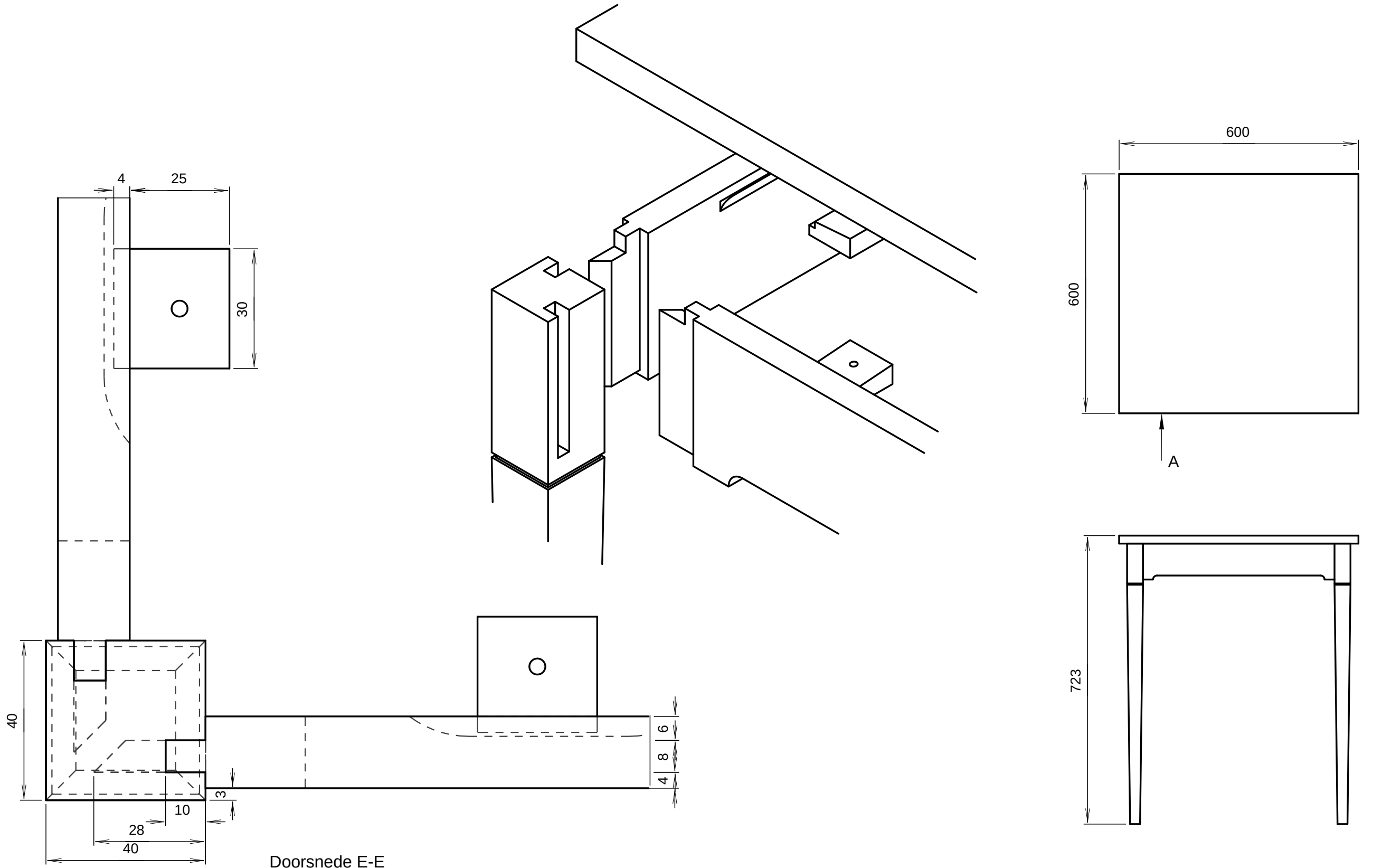
Doorsnede E-E
