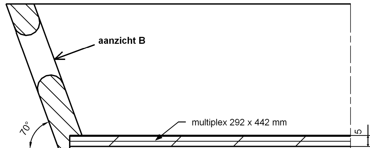
doorsnede A-A
