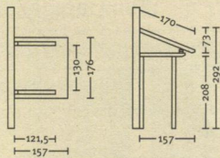
Vordach Wismar Typ 2, Innenansicht
