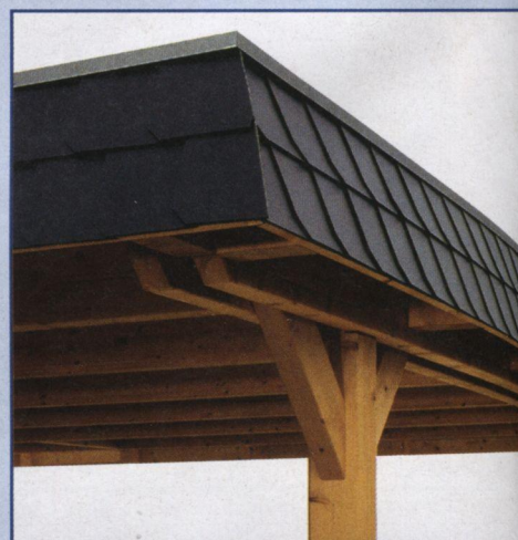
Walmdach: Blende in Schieferoptik mit Aluminiumabschluss; Konstruktion mit Doppelpfette
