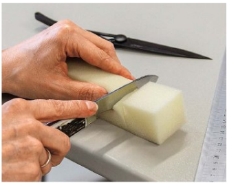
VERGLEICH: An flexiblem Schaumstoff untersuchte die VPA die Schärfe.
