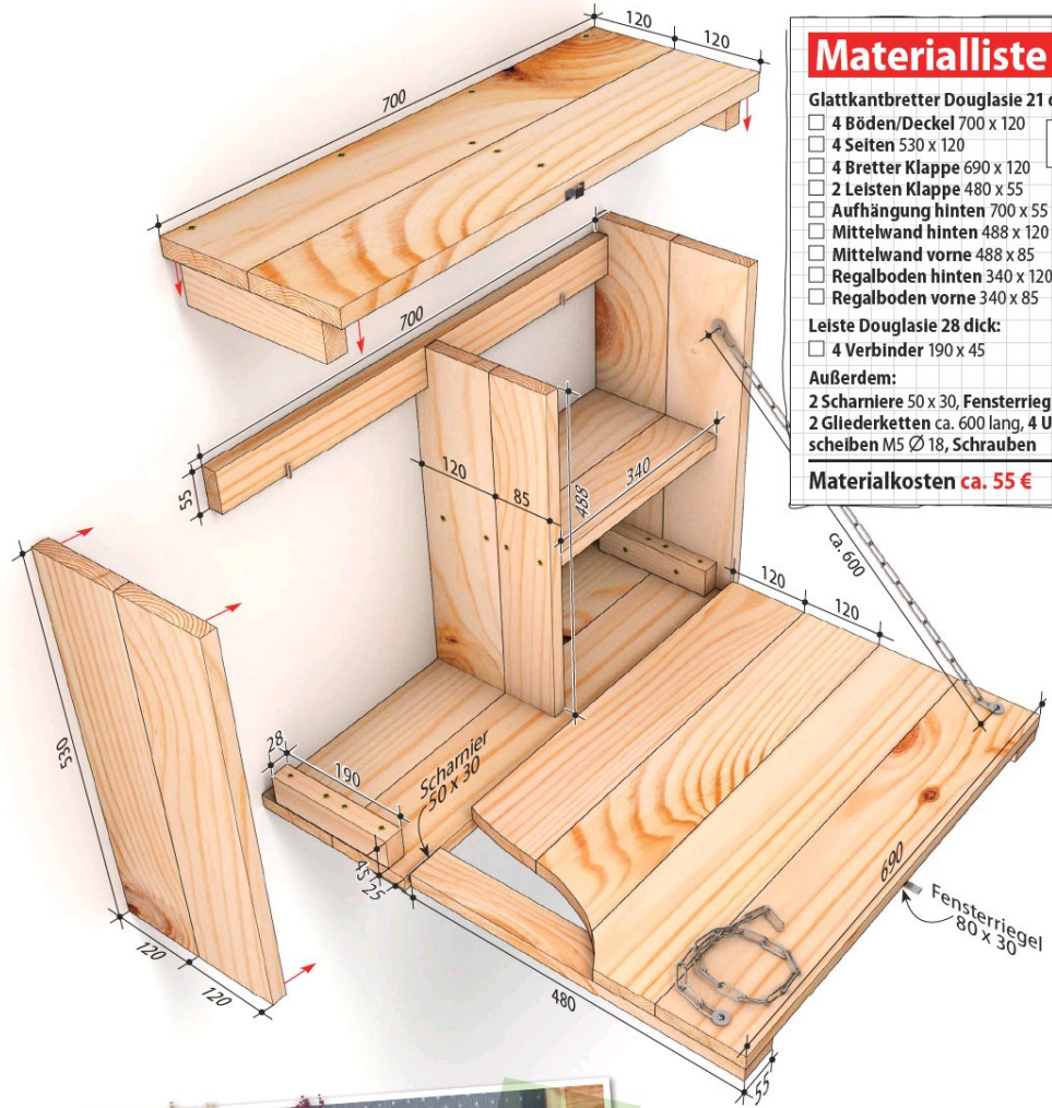
12 Damit die Außenklappe bündig schließt, springt das zweite Brett etwas zurück. Dieses entsprechend auf Breite schneiden.
