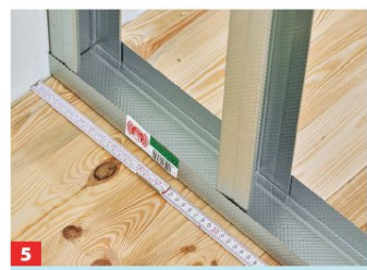
5 Für die Beplankung der 125 cm breiten Platten benötigt man bei Doppelbeplankung einen Achsabstand von 31,25 cm.
