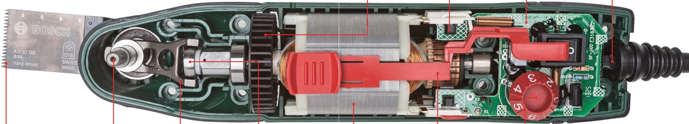
EINSATZWERKZEUG: Die oszillierenden Maschinen waren zuerst als Schleifgeräte etabliert, doch kann man mit ihnen auch exakte Sägeschnitte ausführen – sogar Spachtel- und Raspelarbeiten sind möglich.
