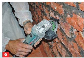
6 ... mit Hammer und Stecheisen oder Winkel- schleifer abtrennen; Löcher vermörteln.
