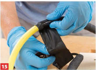
15 Dann wickeln Sie das Vinylband stramm über den Schlauch – zumindest am Anfang und am Ende des Glasfasergewebes.
